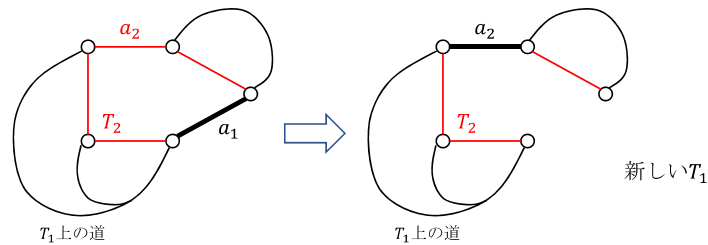
図 10.3.1.2 辺を取り替えて新しい T_1 を作る
