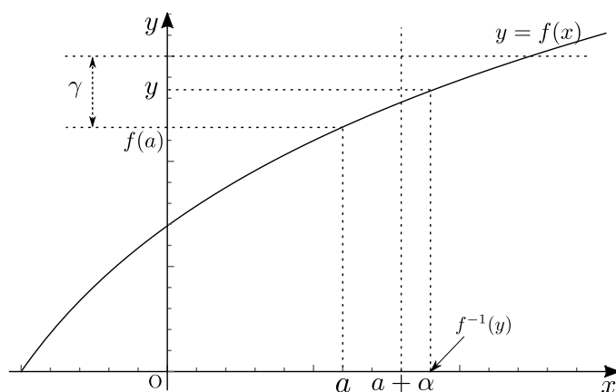
図 5.13.1.1 a, \alpha, \gamma の様子
