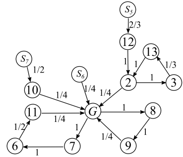
図 XII.4.4 step3
