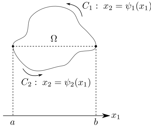
図 III.20.1 積分領域
