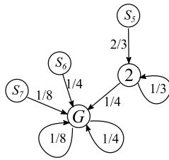
図 9.4.1.5 step4
