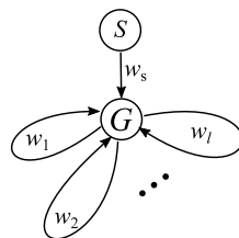
図 9.4.1.7 G(V, E)
