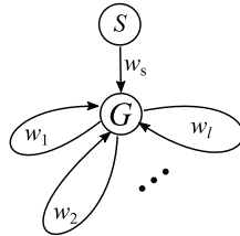
図 9.4.1.8 G(V, E)
