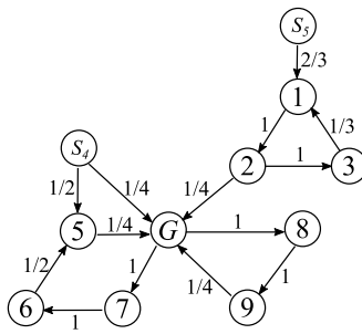
図 9.4.1.2 step1
