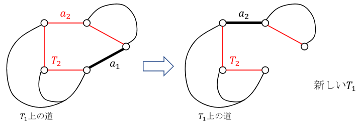
図 9.3.1.2 辺を取り替えて新しい T_1 を作る
