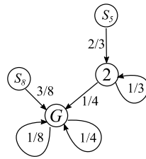
図 9.4.1.6 step5
