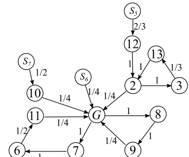
図 9.4.1.4 step3
