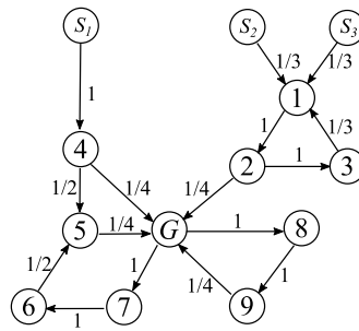
図 9.4.1.1 G(V, E)
