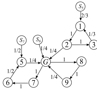
図 9.4.1.3 step2
