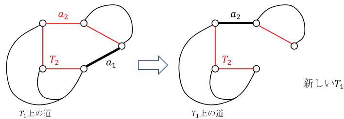
図 9.3.1.2 辺を取り替えて新しい T_1 を作る
