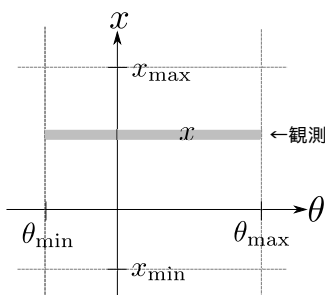
図 XII.1.1 事象 \theta と x の同時確率密度
