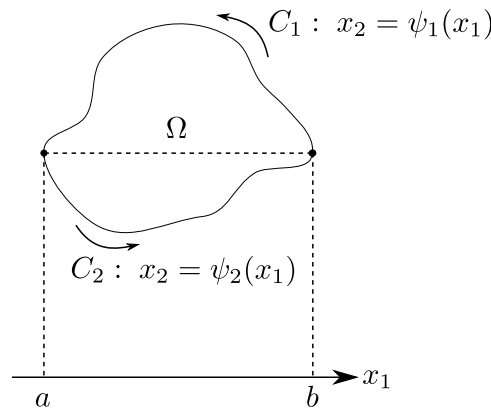
図 3.20.3.1 積分領域
