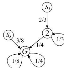
図 10.4.1.6 step5
