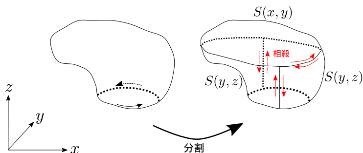
図 8.2.8.1 S の分割
