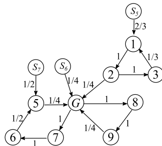
図 10.4.1.3 step2
