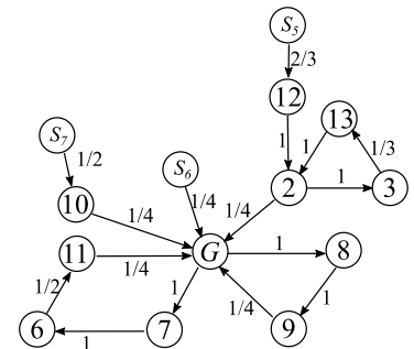
図 10.4.1.4 step3
