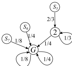
図 10.4.1.5 step4
