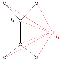
図 10.3.1.1 最小の I_1
