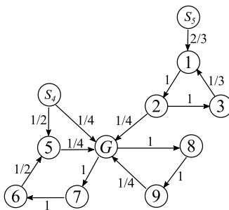
図 10.4.1.2 step1
