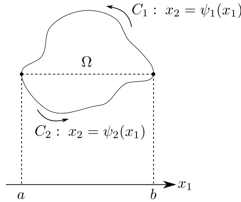
図 5.21.3.1 積分領域
