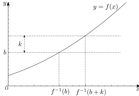
図 5.14.2.1 様子
