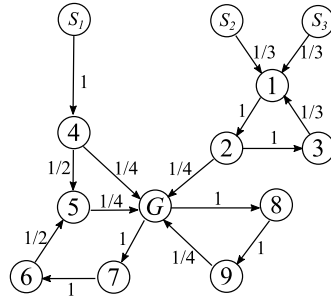
図 10.4.1.1 G(V, E)
