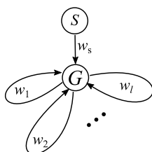
図 10.4.1.7 G(V, E)
