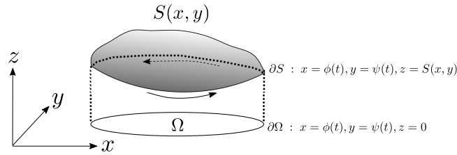
図 8.2.8.2 状況
