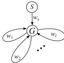
図 10.4.1.8 G(V, E)
