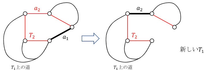
図 XII.3.1 辺を取り替えて新しい T_1 を作る
