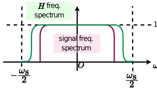
図 7.3.2.1 再標準化前の信号と H の周波数特性
