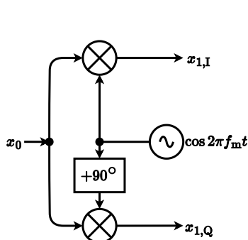
図 11.1.1.1 信号の流れ
