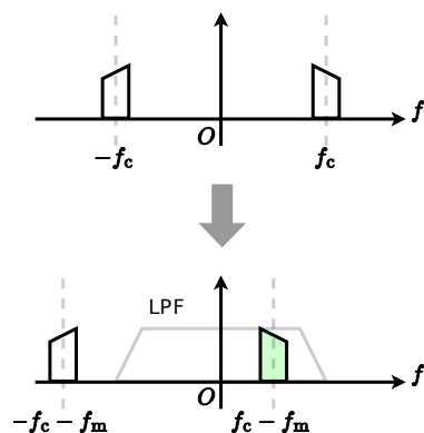
図 11.1.1.2 中間周波信号の周波数スペクトラム
