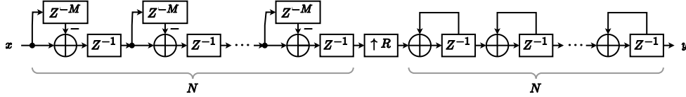
図 13.2.5.1 CIC up-sampler のブロック図
