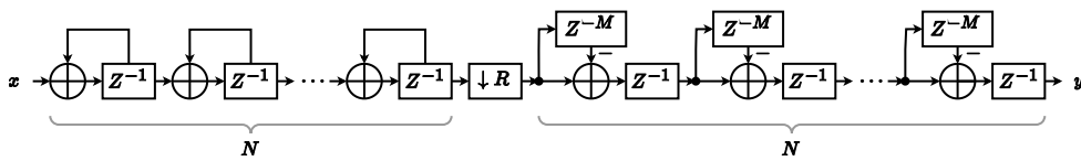
図 13.2.6.1 CIC down-sampler のブロック図
