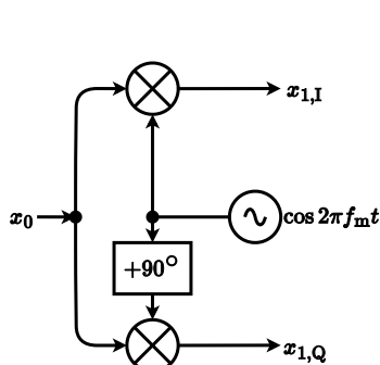
図 11.1.1.1 信号の流れ
