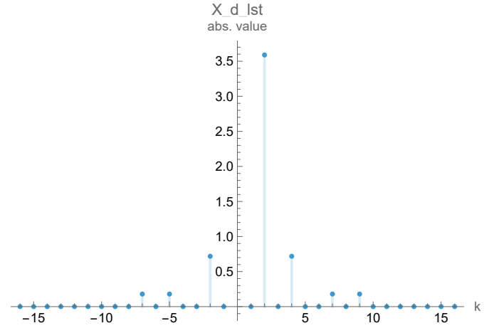
図 12.4.2.5 |X_{DTFT}|
