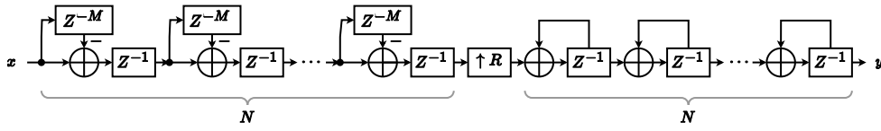
図 13.2.5.1 CIC up-sampler のブロック図
