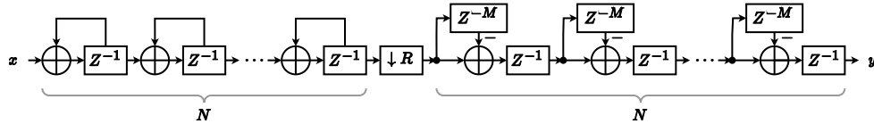
図 13.2.6.1 CIC down-sampler のブロック図
