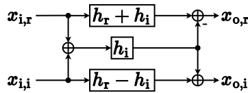
図 13.2.4.1 3 個の feedforward フィルタで実現された系
