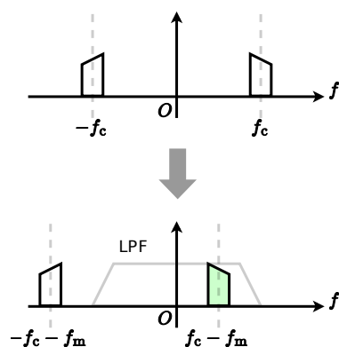
図 11.1.1.2 中間周波信号の周波数スペクトラム
