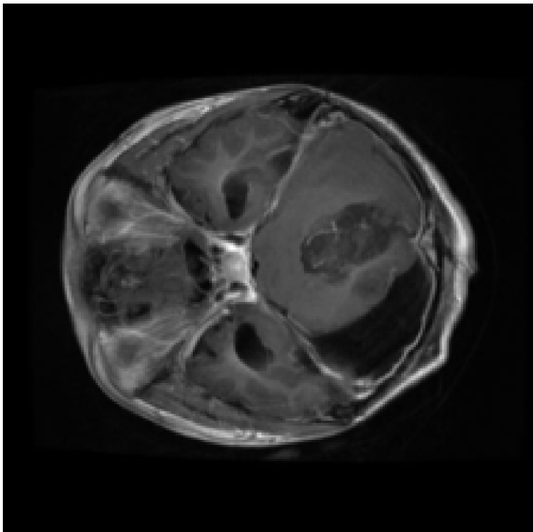
True: Glioma
