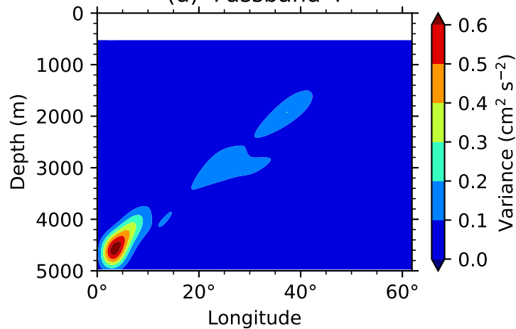
(d) Passband 4
