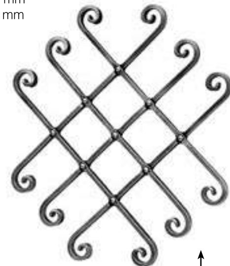
Art. 1657/1 16 x 8 mm 410 mm de Ancho x 400 mm de Alto
