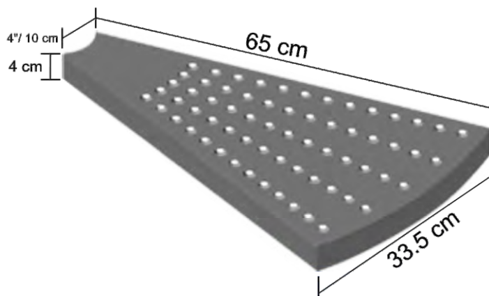
PELDAÑO CARACOL
