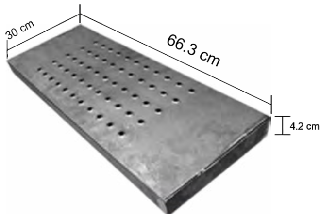
PELDAÑO RECTANGULAR
