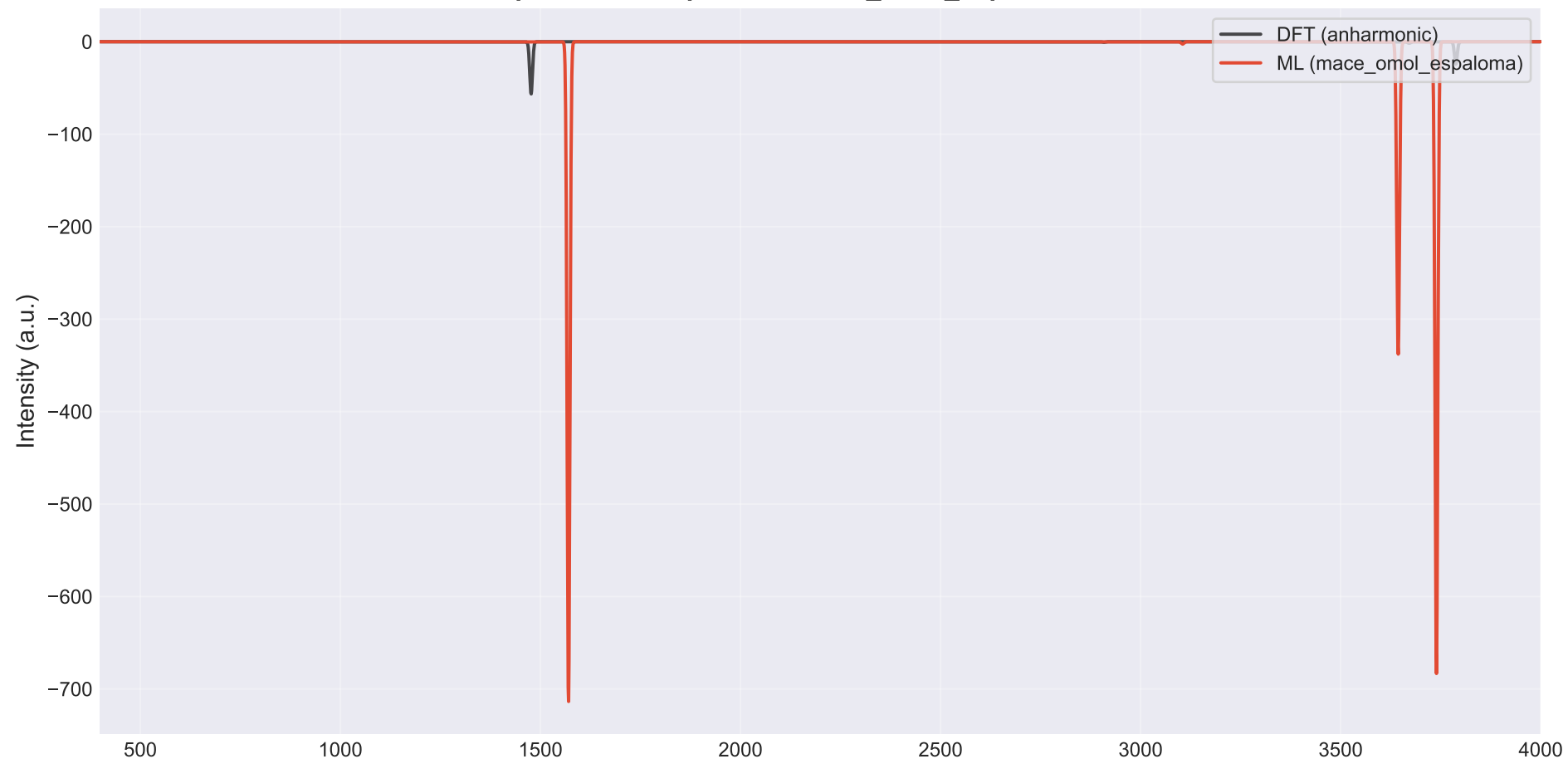
IR Spectrum Comparison: mace_omol_espaloma vs DFT
