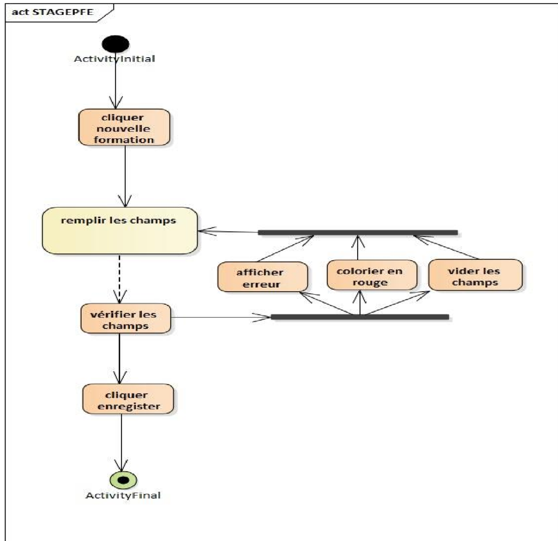
Figure 4 : Diagramme d'activités (Ajout d'une formation)
