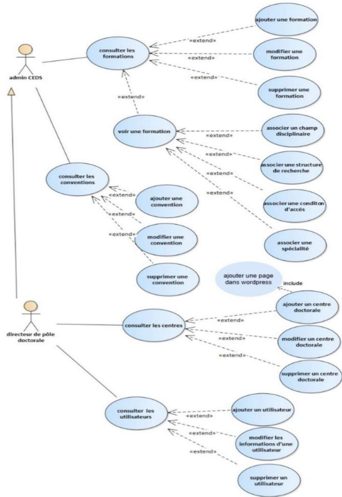
Figure 3 :Diagramme de cas d'utilisation (Administrateur CED et Directeur du Pôle)
