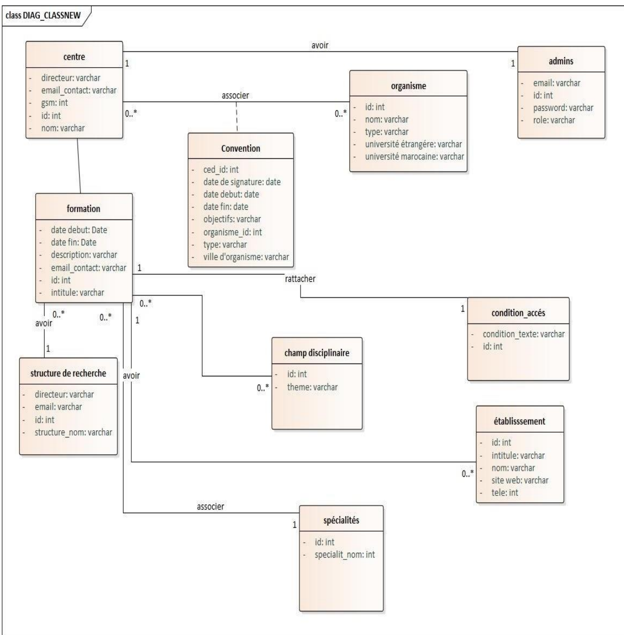
Figure 6 : Diagramme de classe
