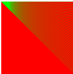
Octant 1 : 400 × 400, fond rouge, de (0, 0) vers (399, y), y de 10 en 10.
