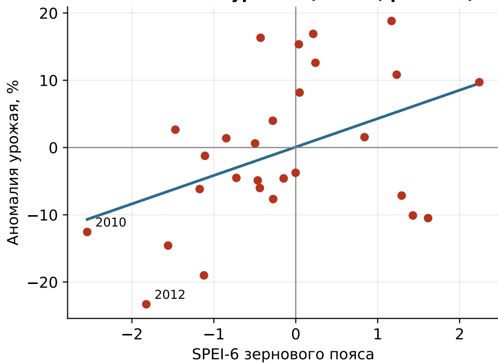
Пояс: SPEI-6 и урожай ( r=0.43 , p=0.022 )
