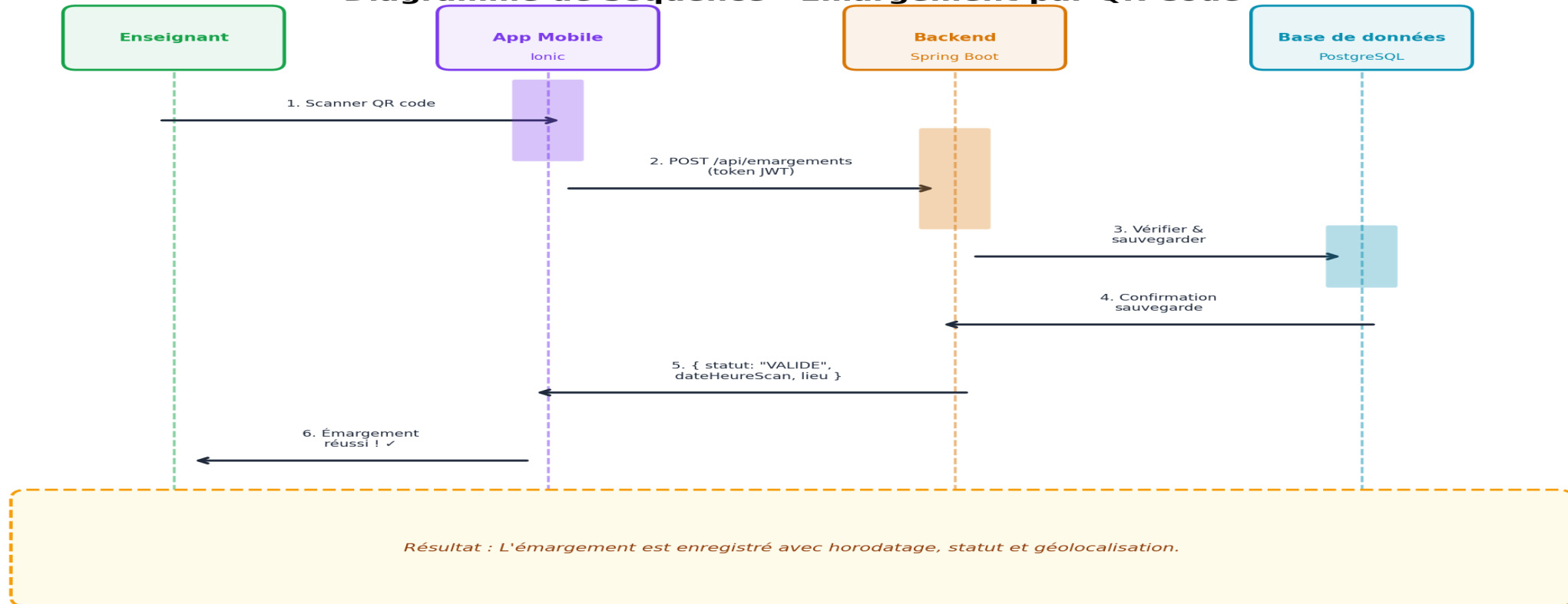
Diagramme de séquence - Émargement par QR Code
