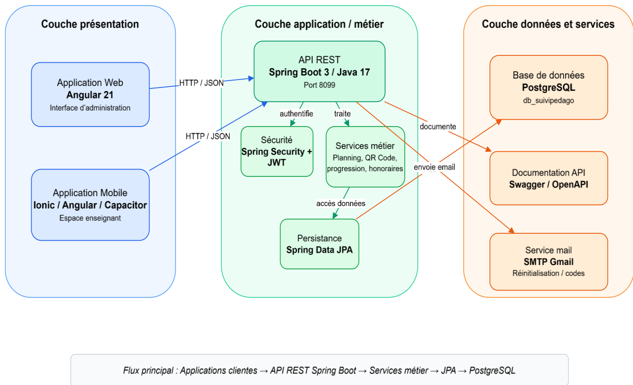
Figure 6: Architecture en trois couches du système EduTrack.
