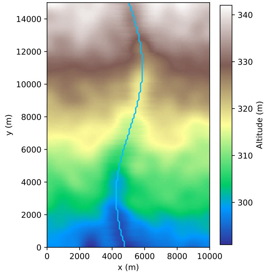
Altitude de la surface (sommet de la couche 1)
