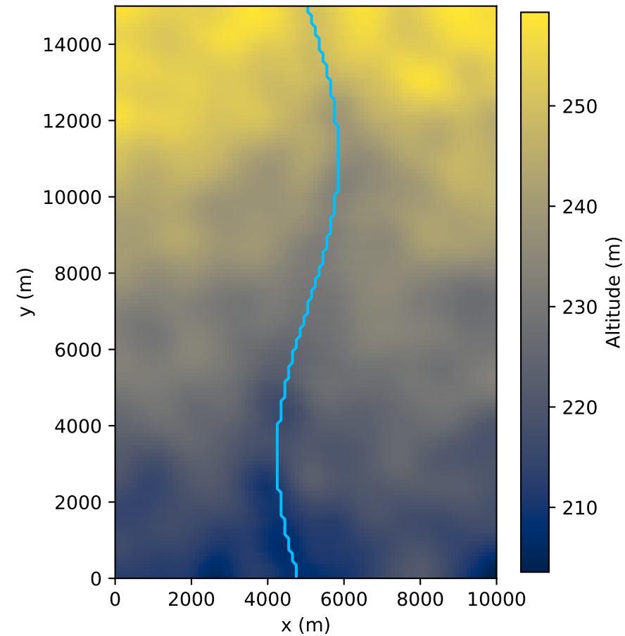
Base du modèle (fond de la couche 3)
