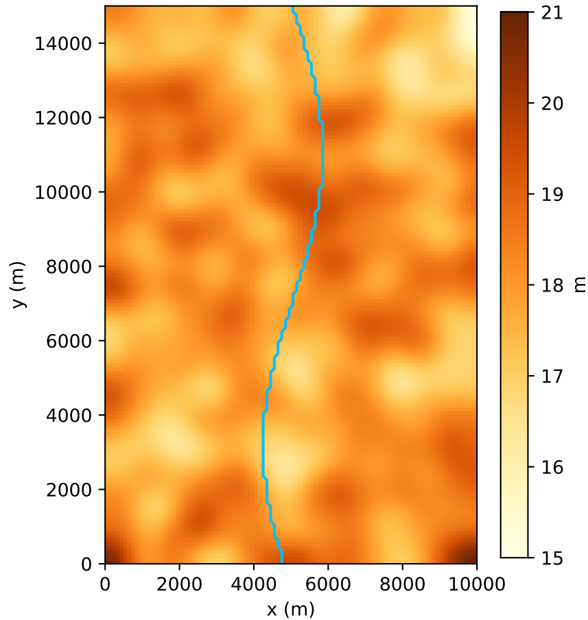
Épaisseur de la couche 1
