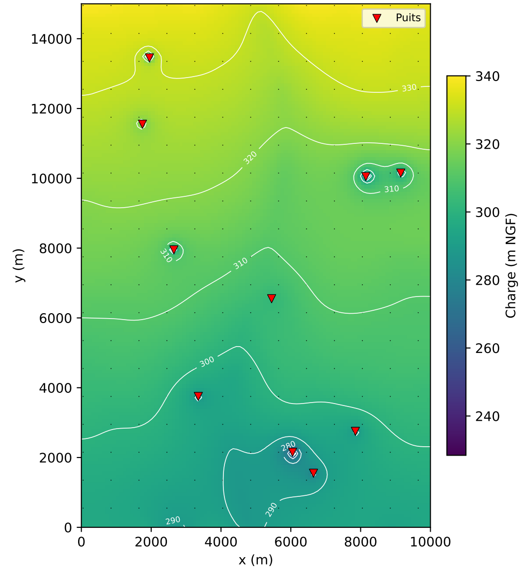
Modèle complet — charge, couche 3
