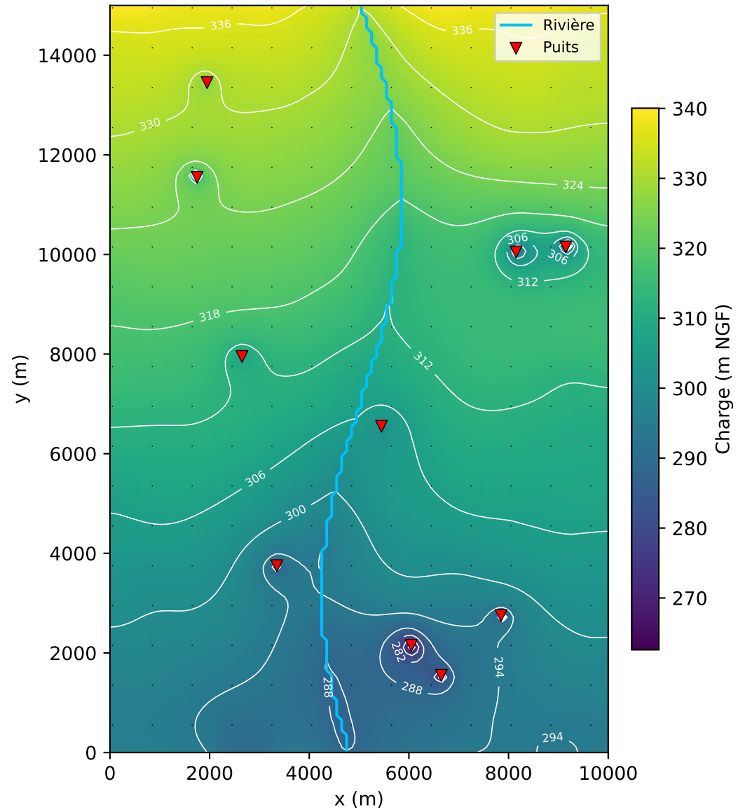
Modèle complet — charge, couche 1
