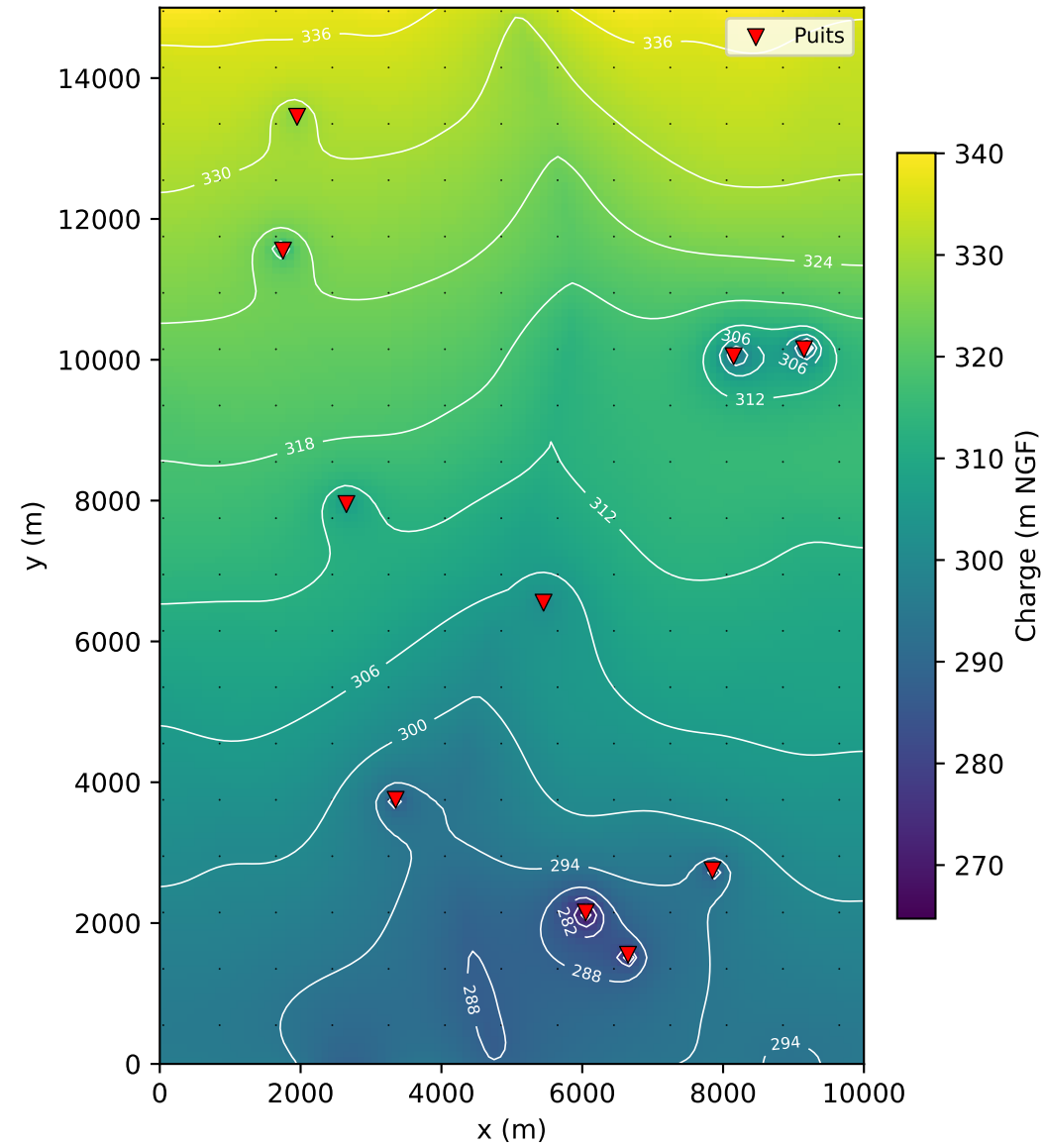
Modèle complet — charge, couche 2
