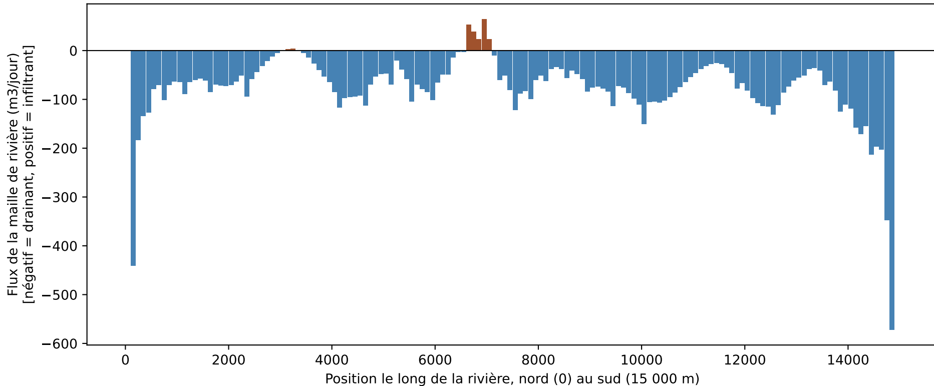
Gains et pertes le long de la rivière (régime permanent, modèle complet)
