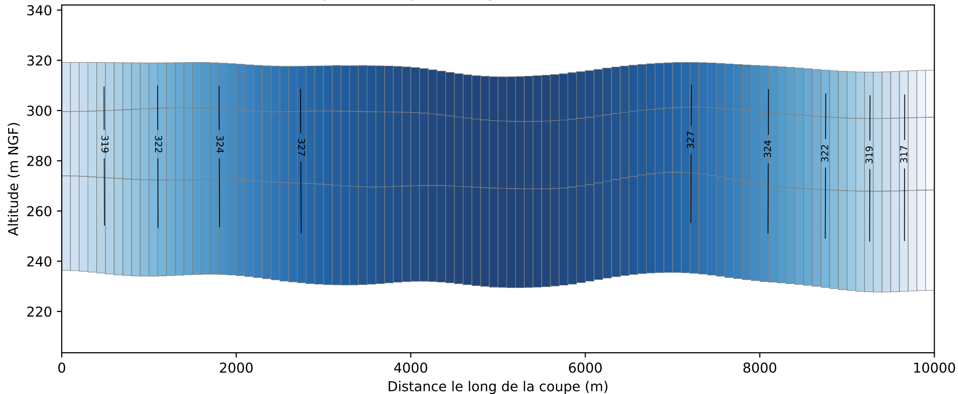
Modèle de base (étape 2) : coupe E-O (ligne 75) -- notez le monticule dans la vallée
