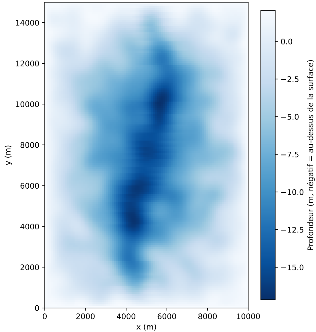
Profondeur de la nappe (charges de l'étape 2)
