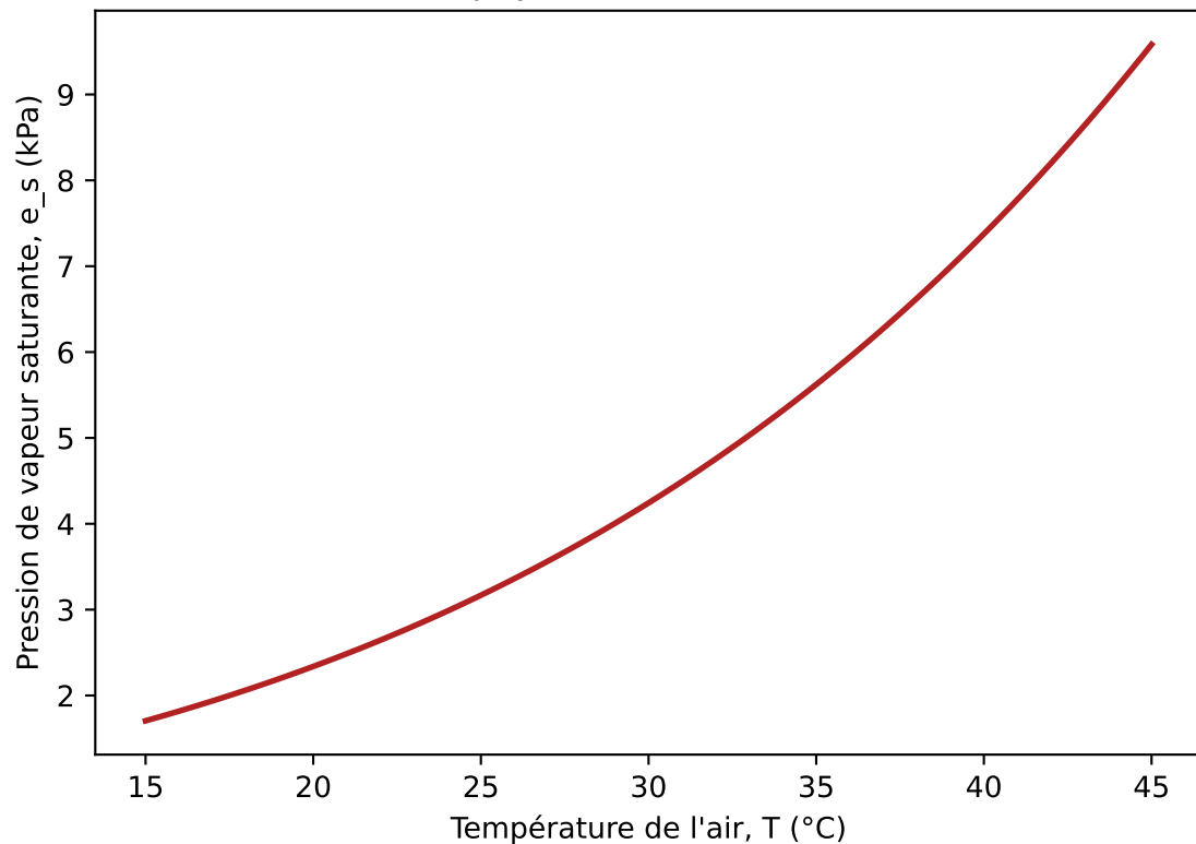
Loi de Clausius-Clapeyron : croissance non linéaire avec T
