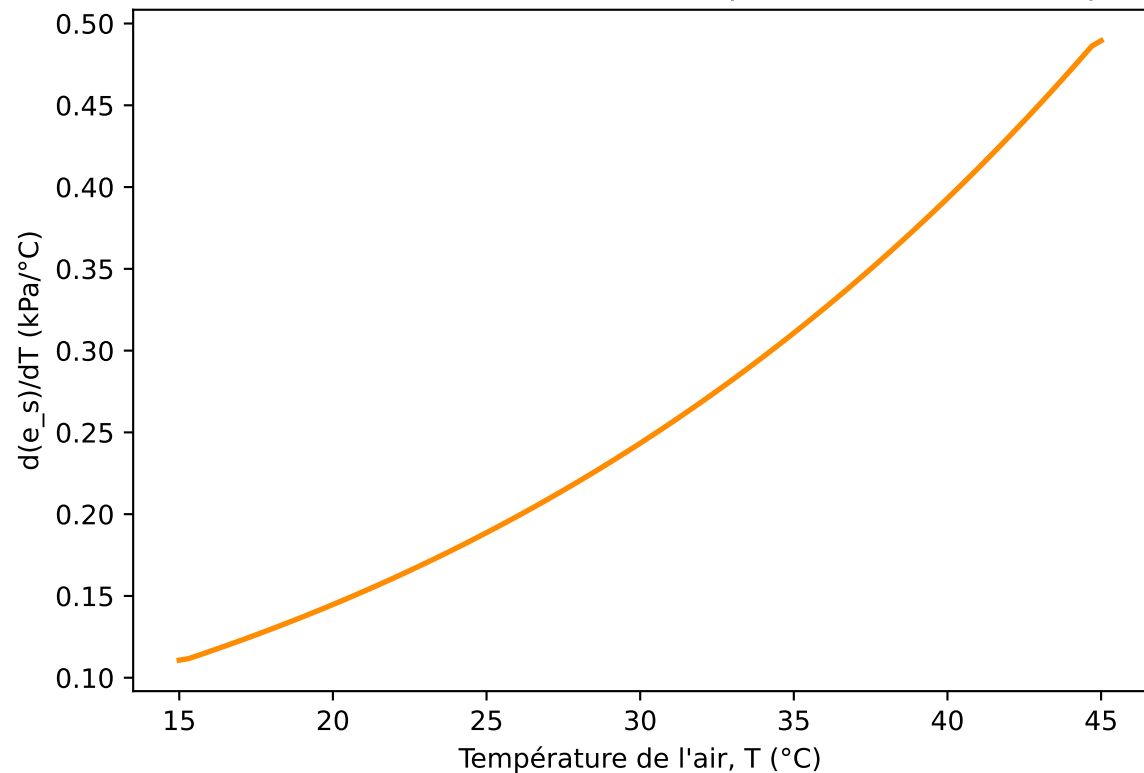
Sensibilité de l'ETP à un réchauffement -- plus forte à haute température
