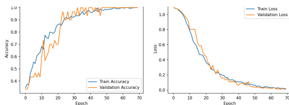
figure 7: variation de Accuracy et loss en fonction de epoch
