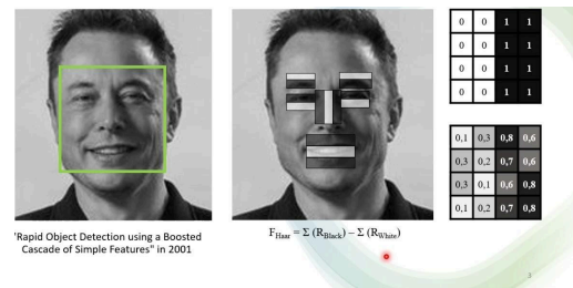
figure 6: caractéristiques Haar
