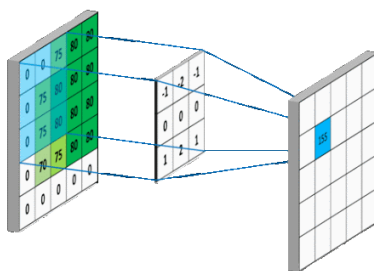
figure 5: extraction des caractéristiques
