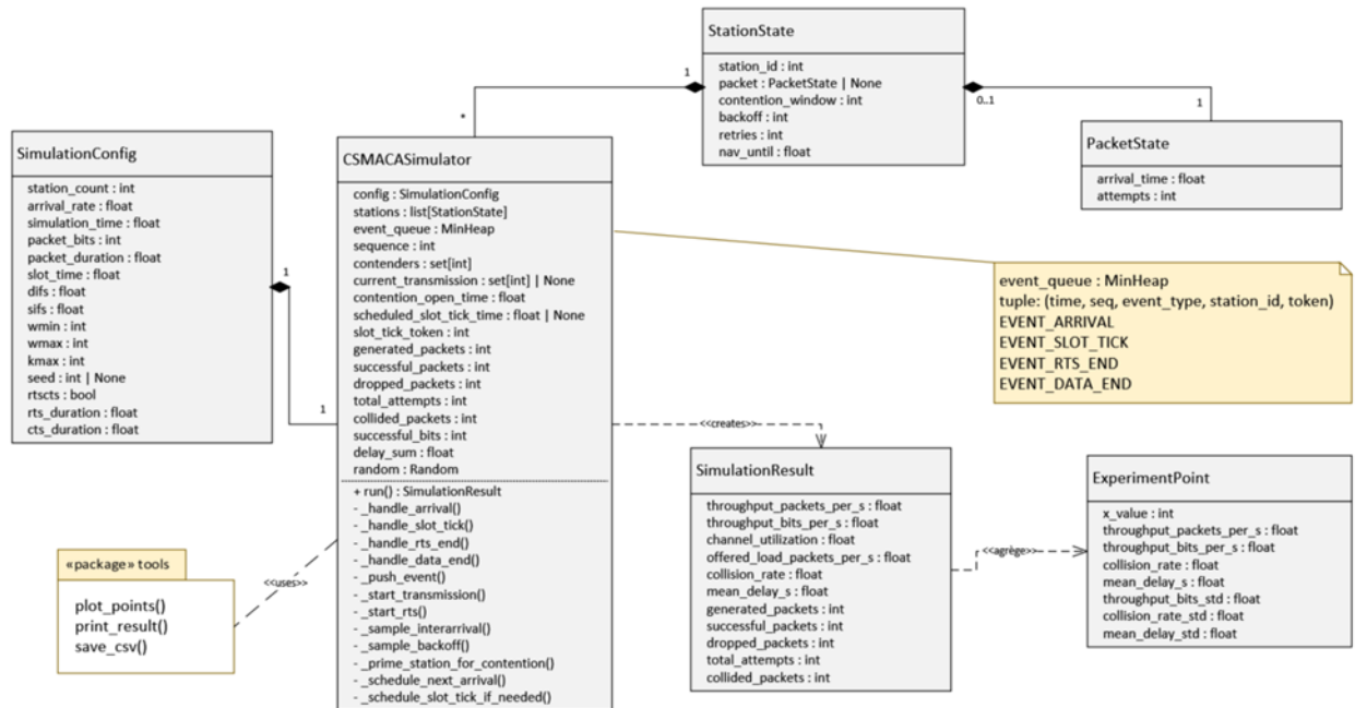
Figure 2 — Diagramme de classes UML du simulateur CSMA/CA
