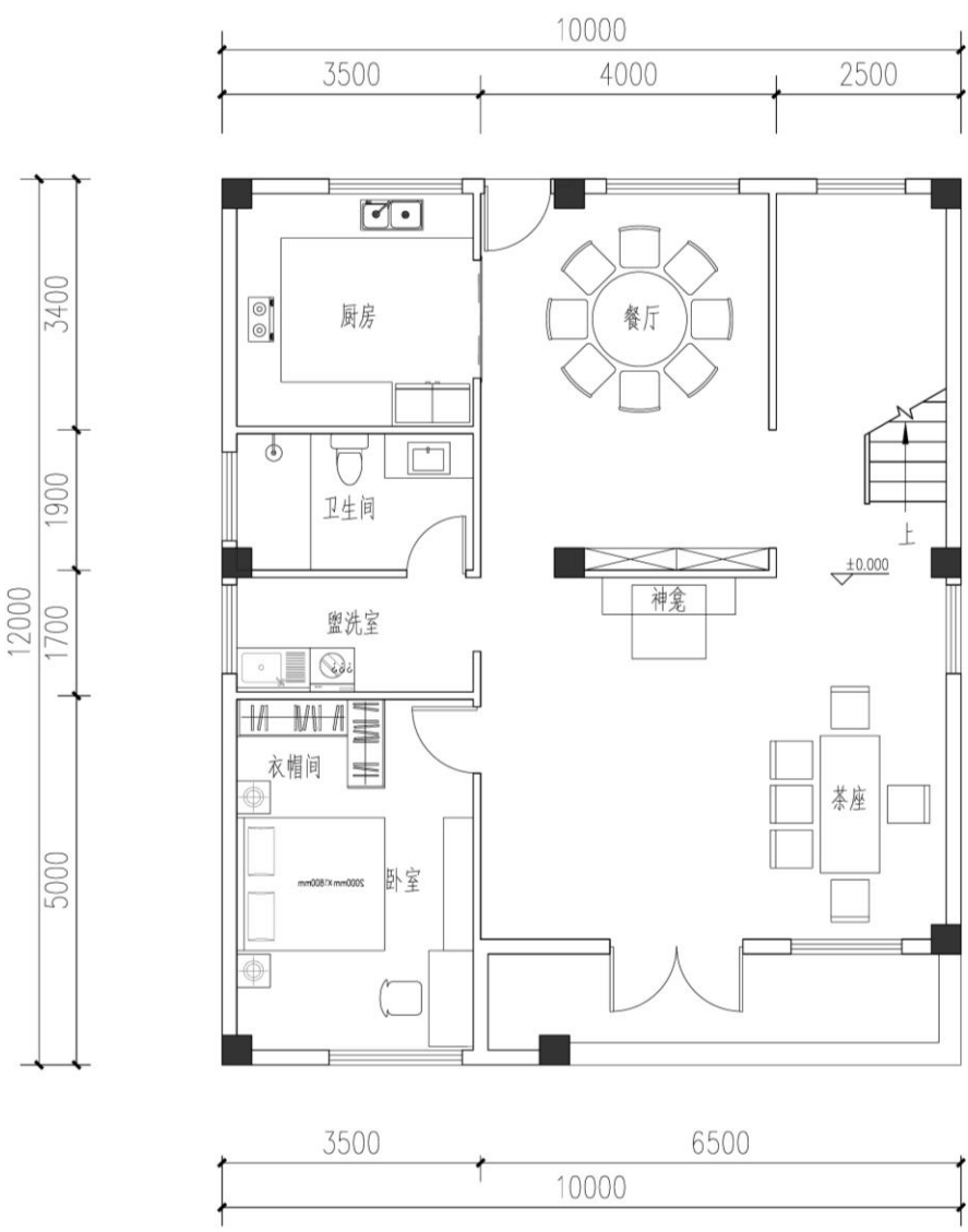
首层平面图
