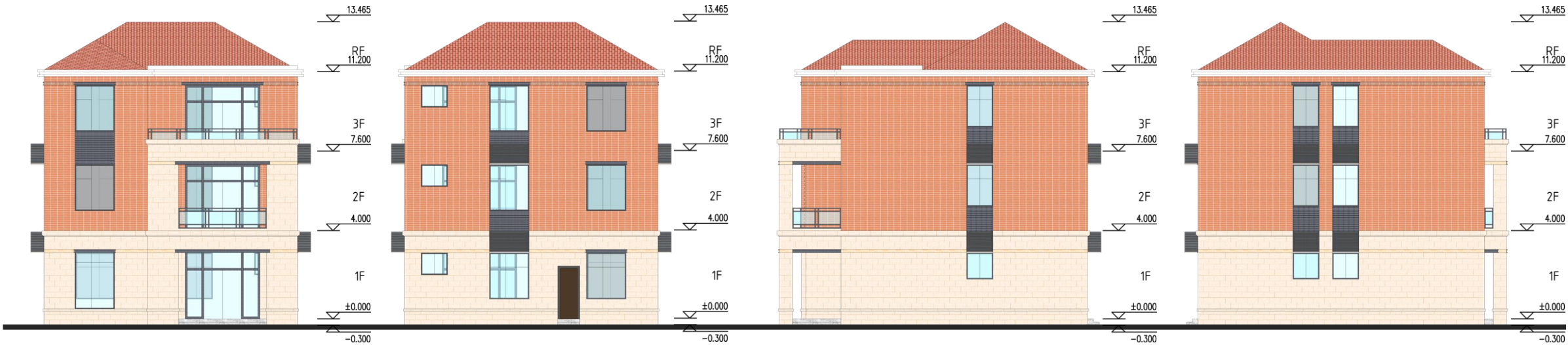
正向立面
