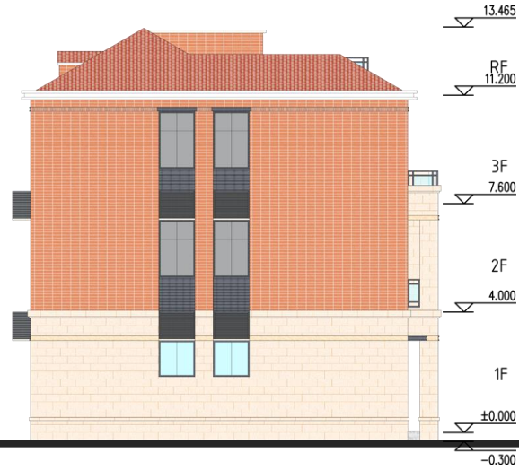
左侧立面
