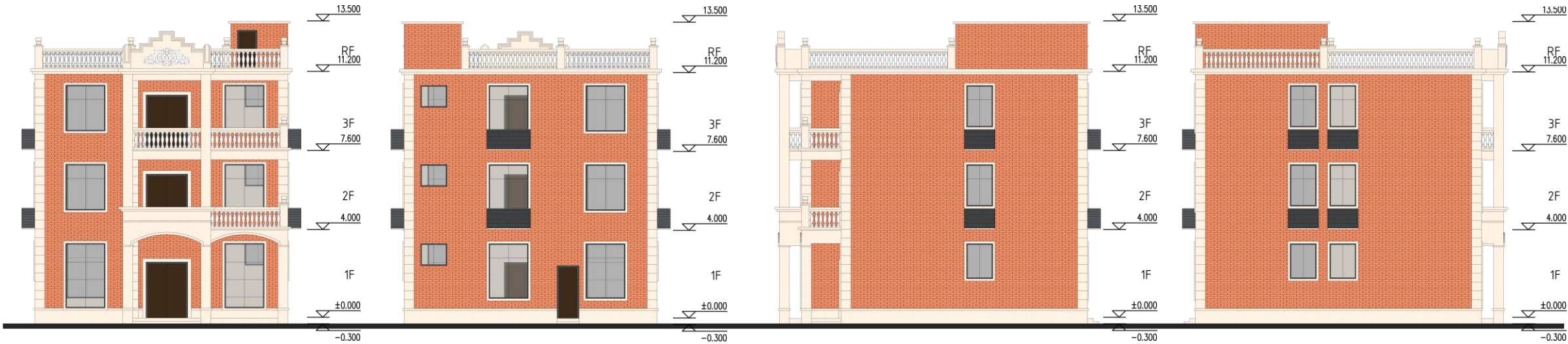
正向立面
