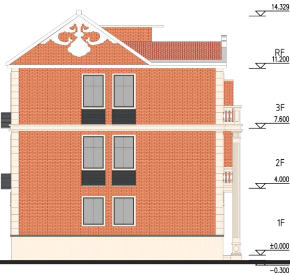
左侧立面
