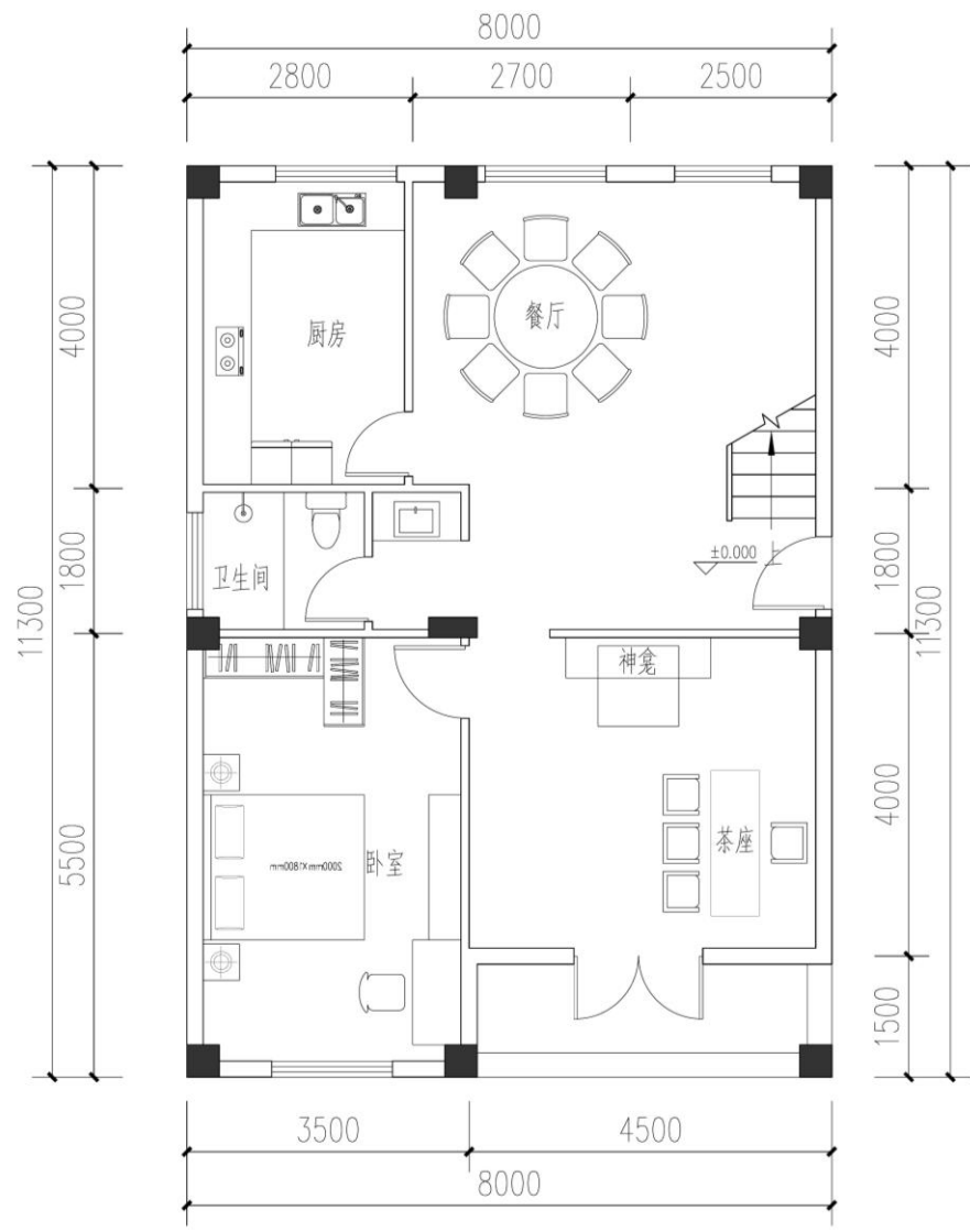
首层平面图
