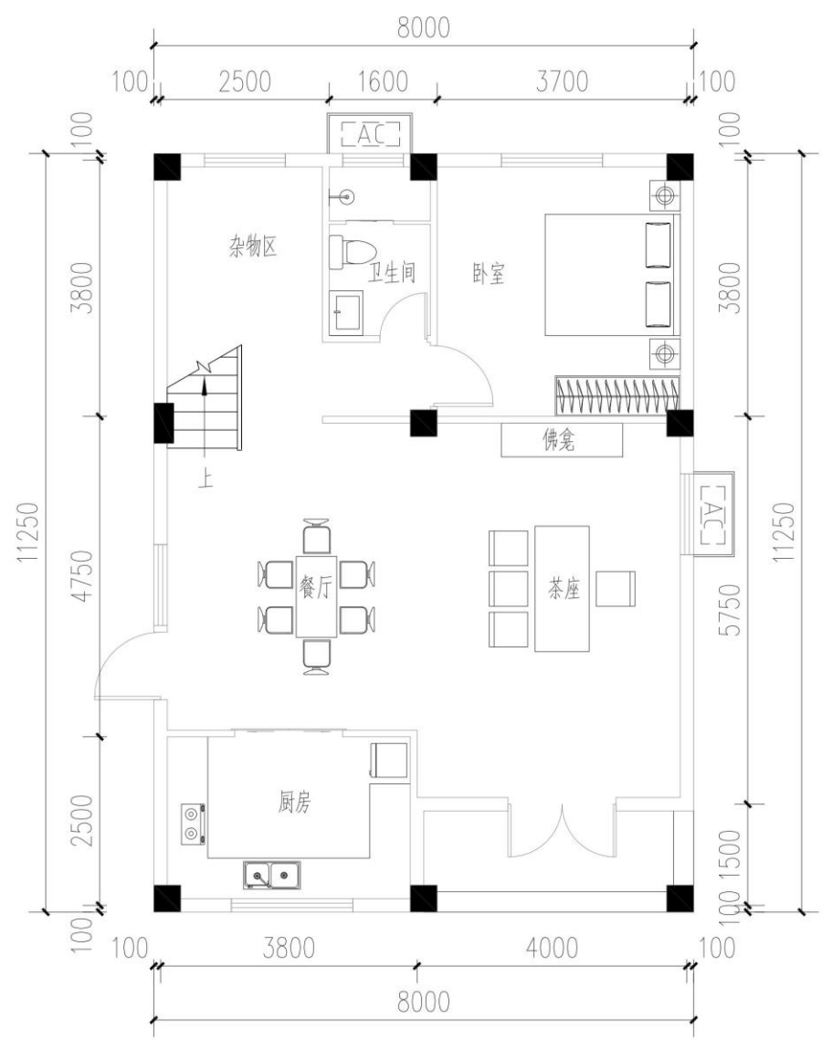
首层平面图
