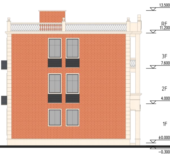
左侧立面
