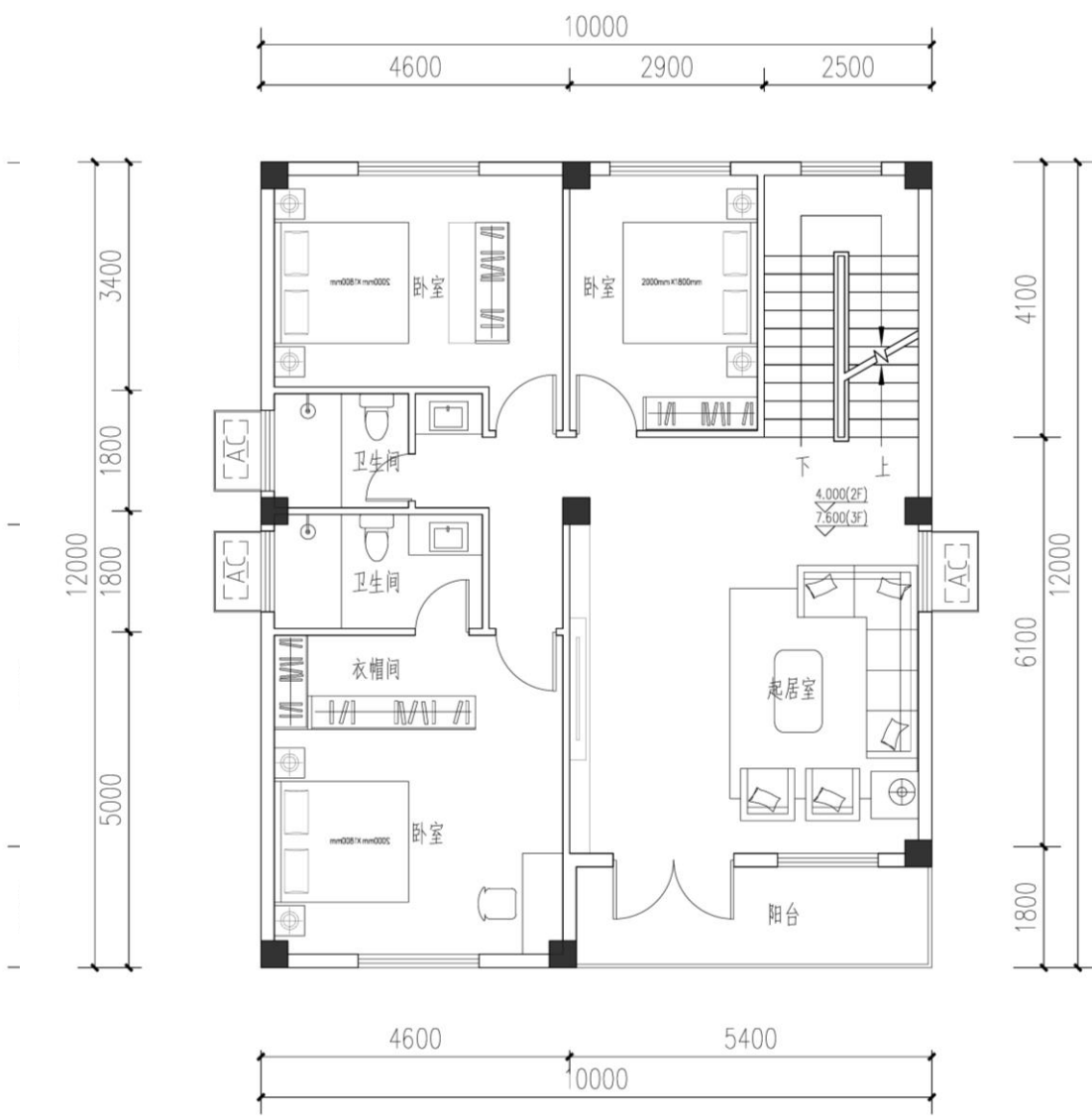
二、三层平面图
