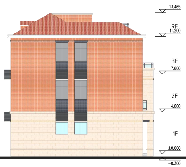
左侧立面
