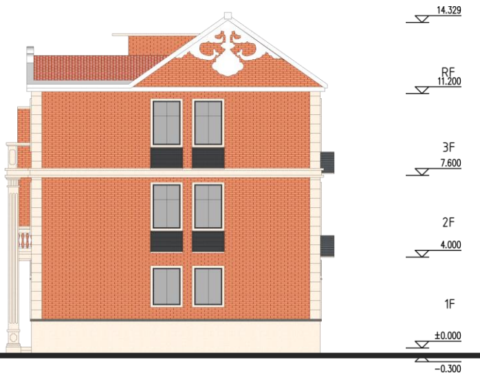
背向立面
