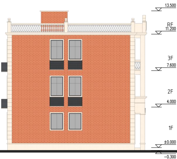
左侧立面
