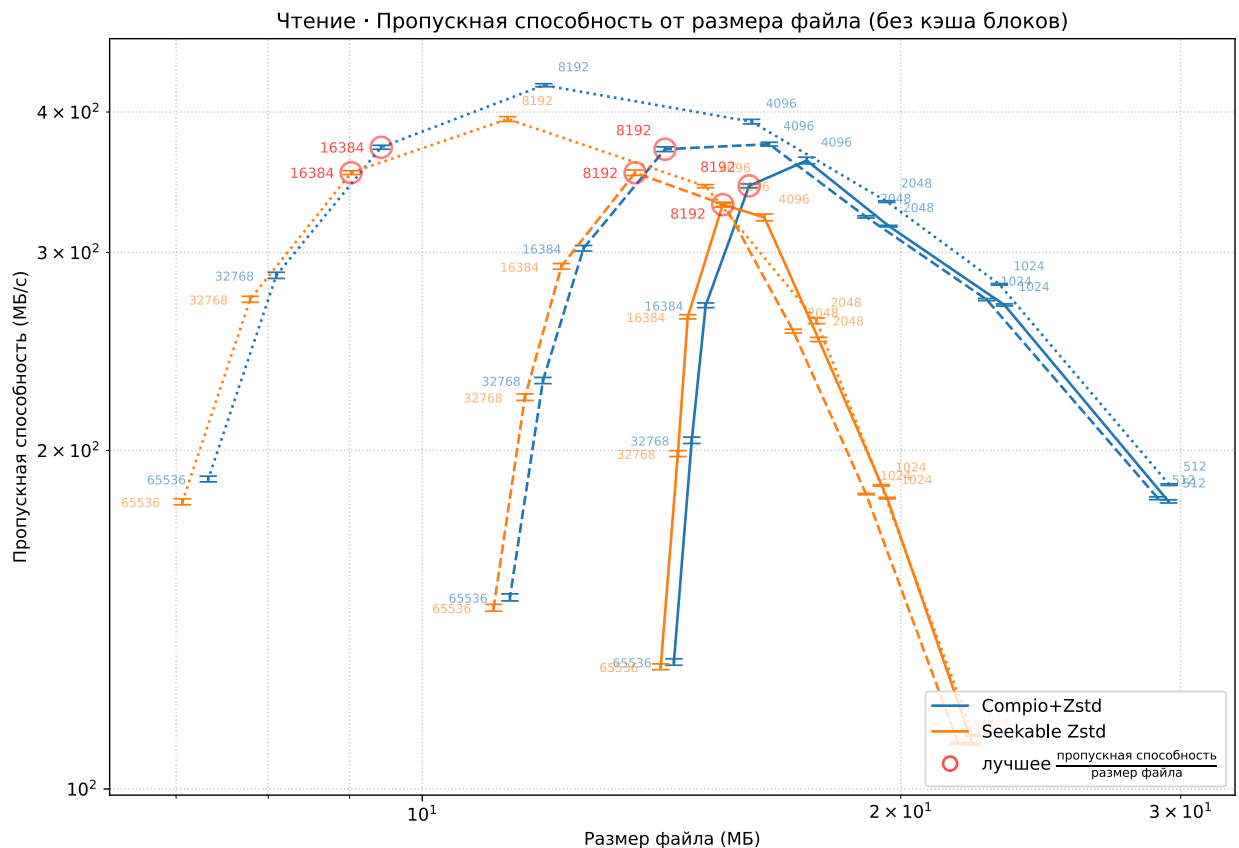
Рис. 5: Сравнение Compio (Zstd, уровень 1) и Seekable Zstd на трёх участках enwik9[18]. Инструменты различаются цветом, участки — стилем линии. Точки — разные параметры гранулярности. Красные кружки — максимум отношения скорости к размеру архива. В области своих оптимальных для данного сценария использования параметров гранулярности (8–16 КиБ) инструменты практически идентичны.
