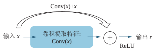
图 3 残差连接
