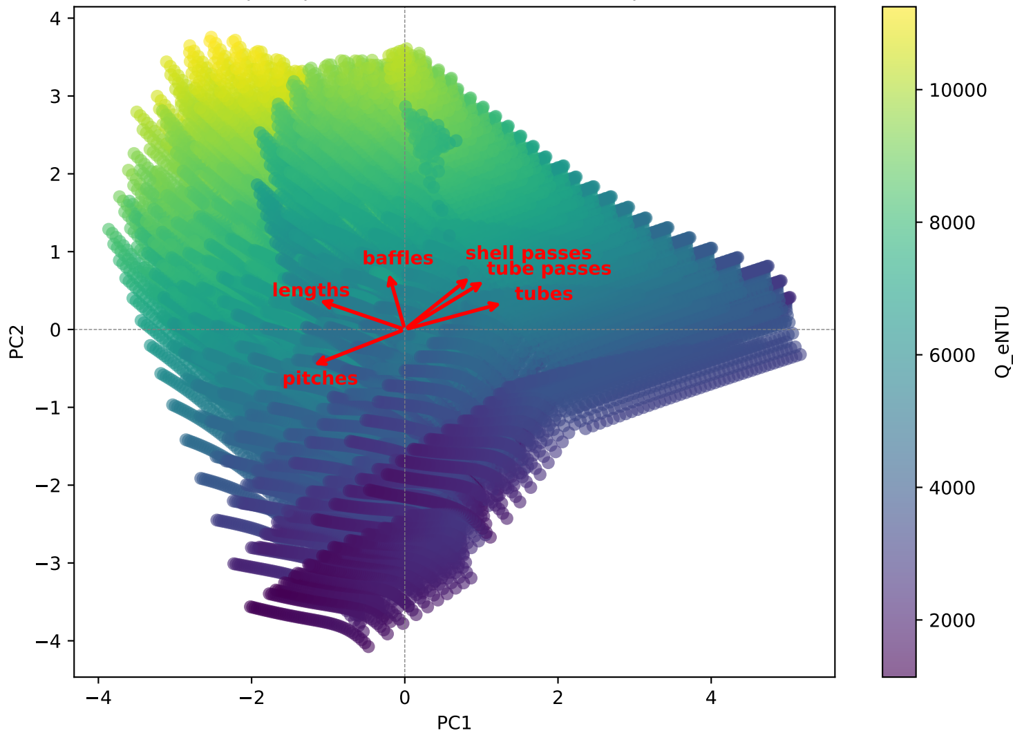
Biplot: parameter directions in PCA space
