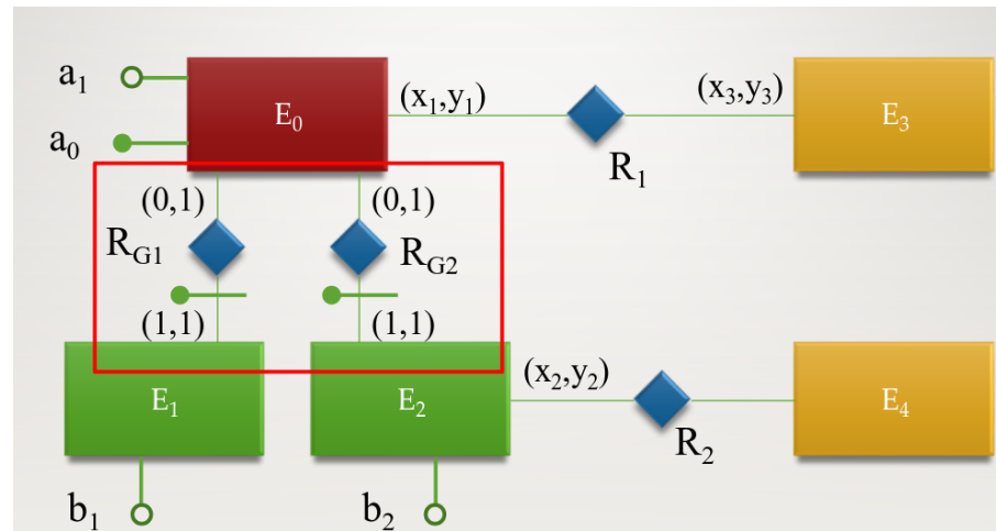
Figura 38: Esempio dopo l'accoppiamento di entità e relazioni
