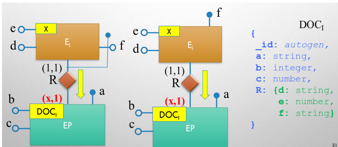
Figura 70: Regola di traduzione per entità principale con entità debole
