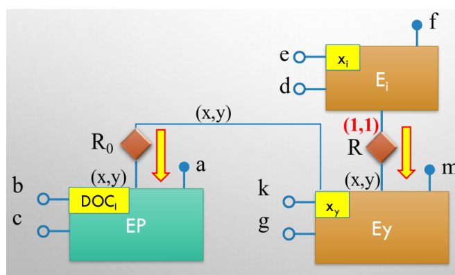
Figura 63: Esempio di incapsulamento in un'entità non principale
