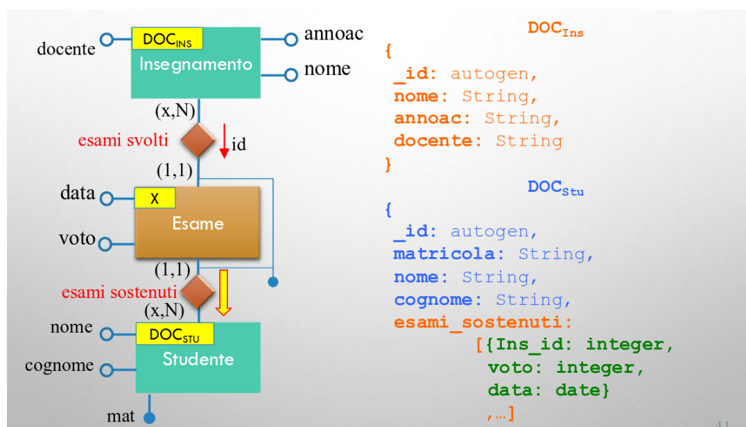
Figura 79: Esempio di traduzione di relazione binaria tra entità non principale ed entità principale
