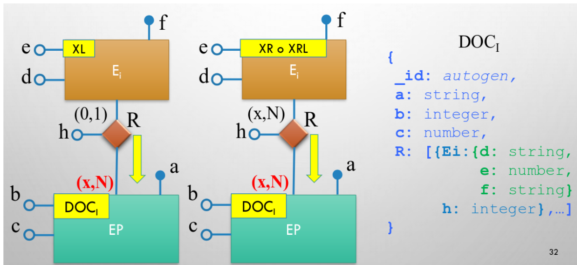
Figura 71: Regola di traduzione per entità principale con entità debole
