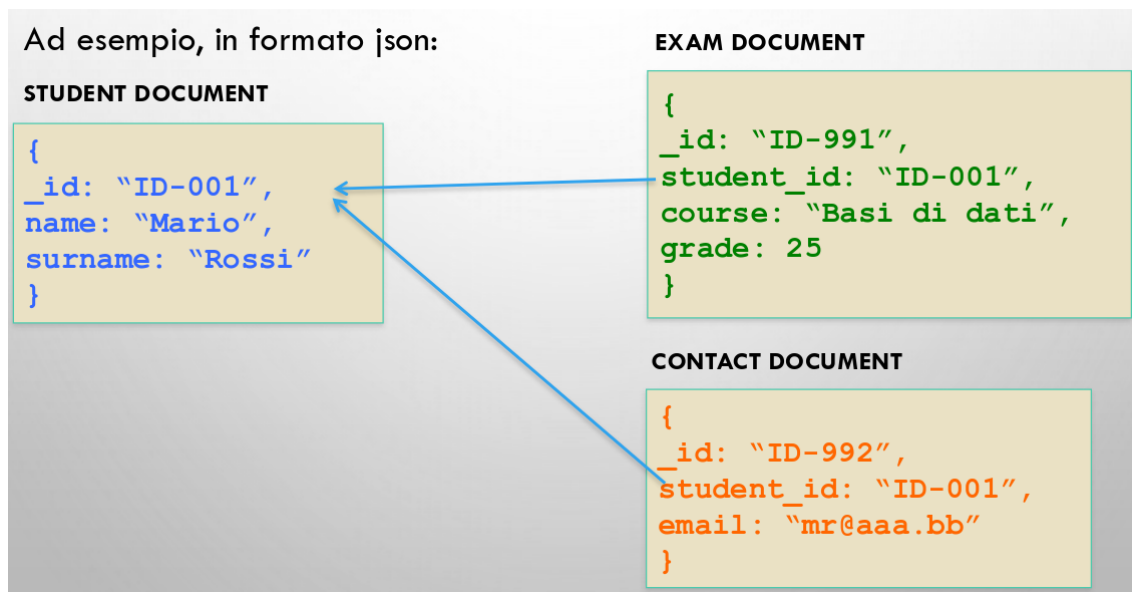
Figura 53: Esempio di documenti con riferimenti
