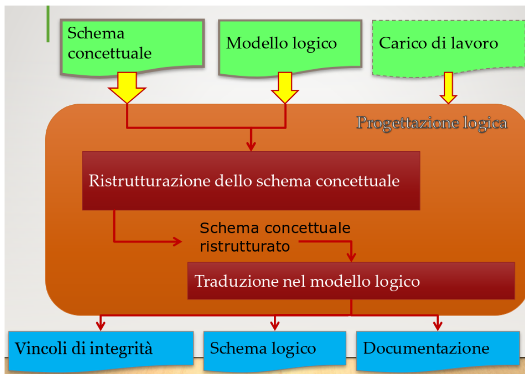
Figura 32: Diagramma della progettazione logica
