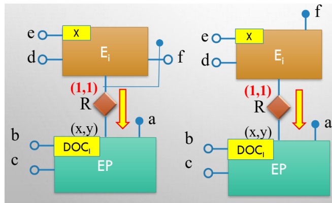
Figura 59: Esempio di incapsulamento con cardinalità (1,1)
