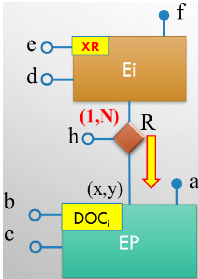
Figura 61: Esempio di incapsulamento con cardinalità (1,N)
