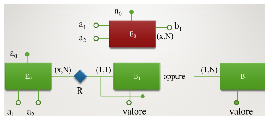
Figura 40: Esempio dopo il partizionamento dell'entità
