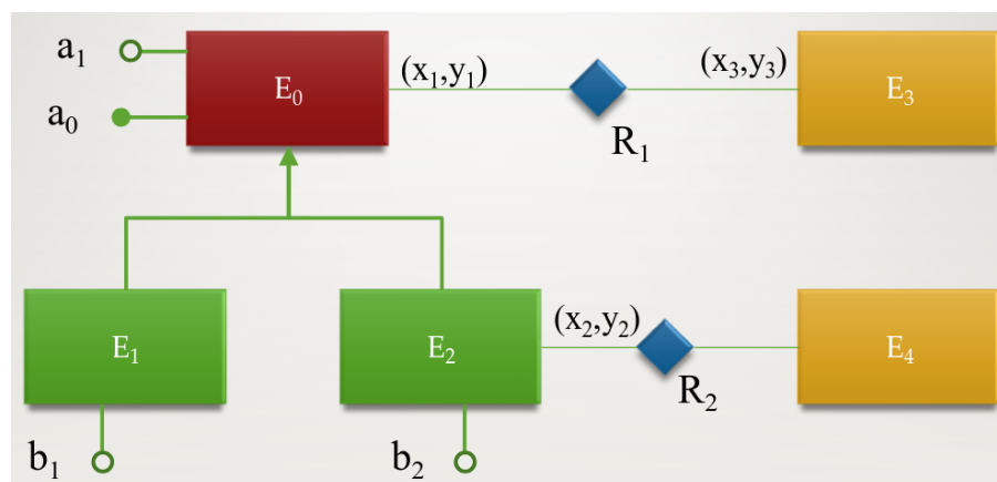
Figura 37: Esempio di accorpamento di entità e relazioni
