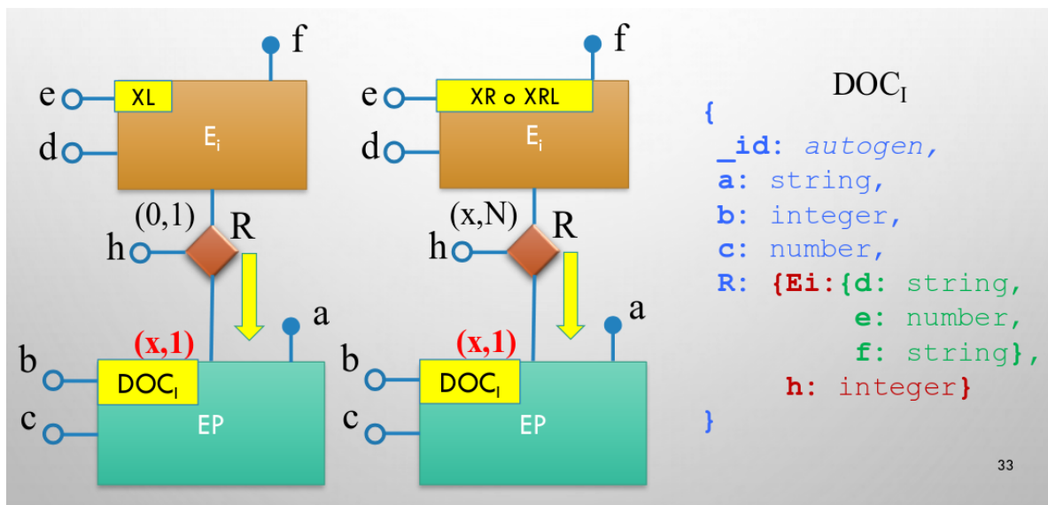
Figura 72: Regola di traduzione per entità principale con entità debole
