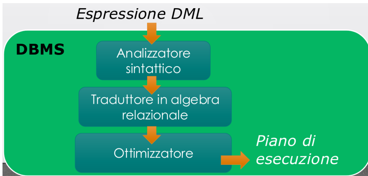
Figura 84: Ottimizzazione di espressioni DML
