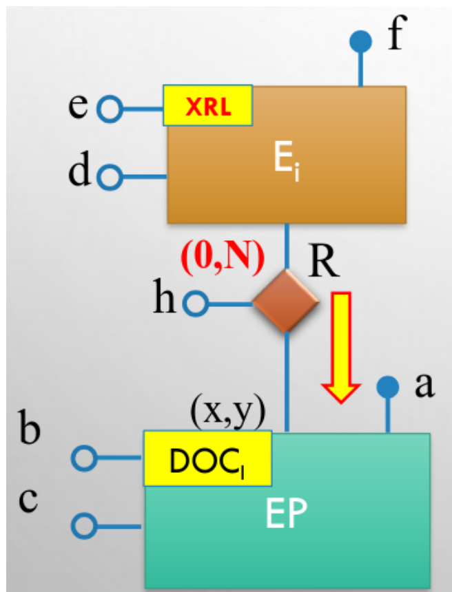
Figura 62: Esempio di incapsulamento con cardinalità (0,N)
