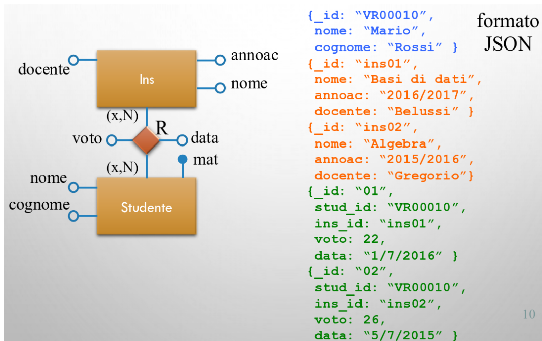
Figura 55: Esempio di documenti normalizzati
