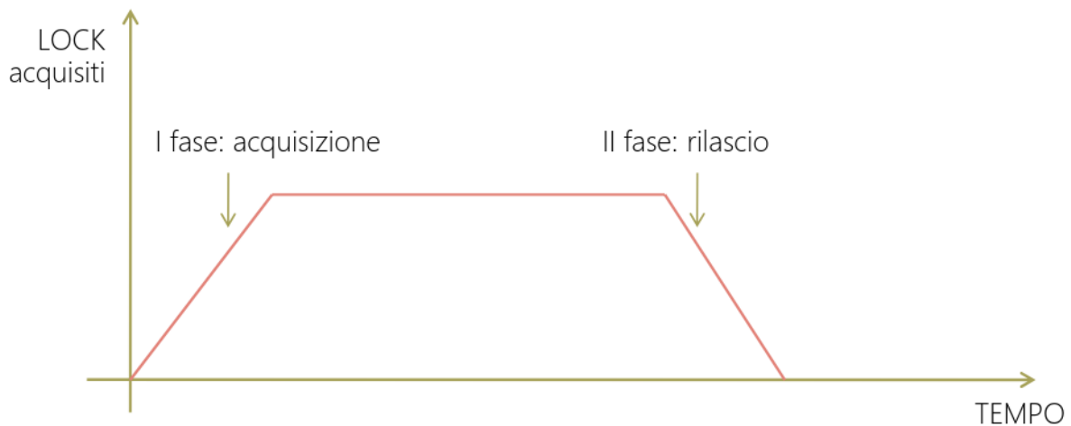
Figura 62: Locking a due fasi
