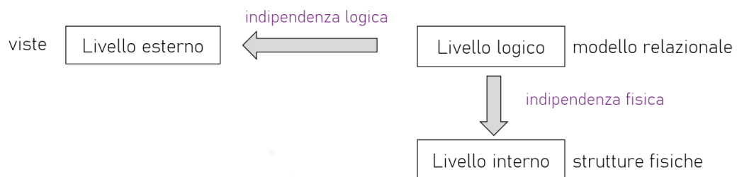
Figura 1: Architettura a 3 livelli di un DBMS
