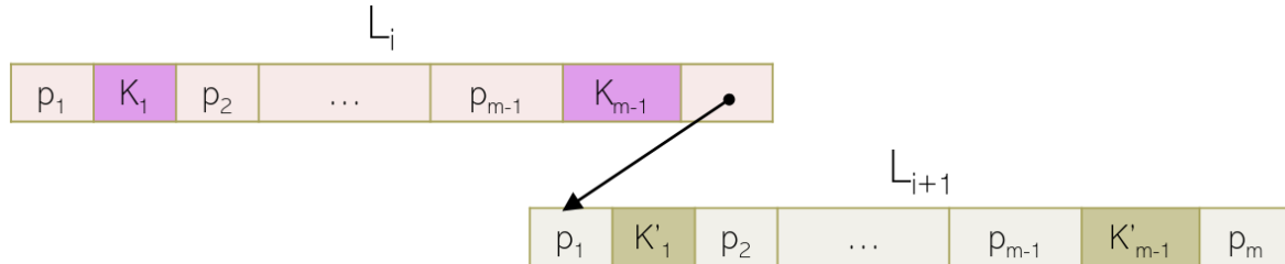
Figura 44: Puntatore p_m del nodo L_i che punta al nodo L_{i+1}
