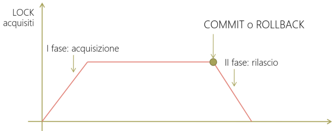
Figura 63: Locking a due fasi stretto
