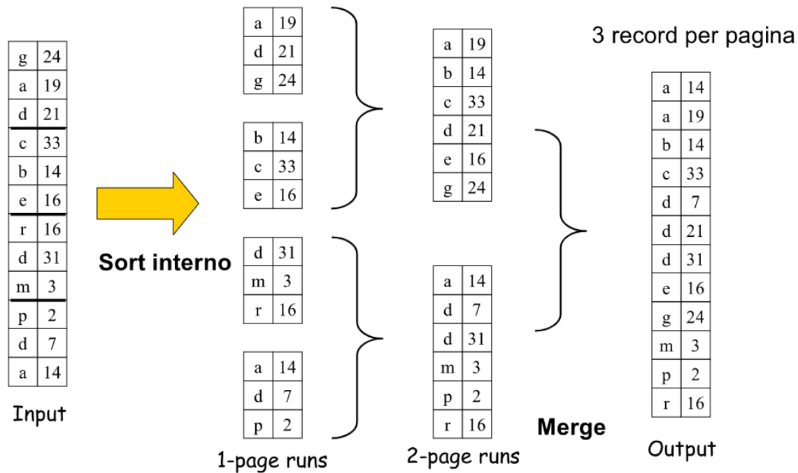
Figura 67: Esempio di ordinamento con Z-way Sort-Merge
