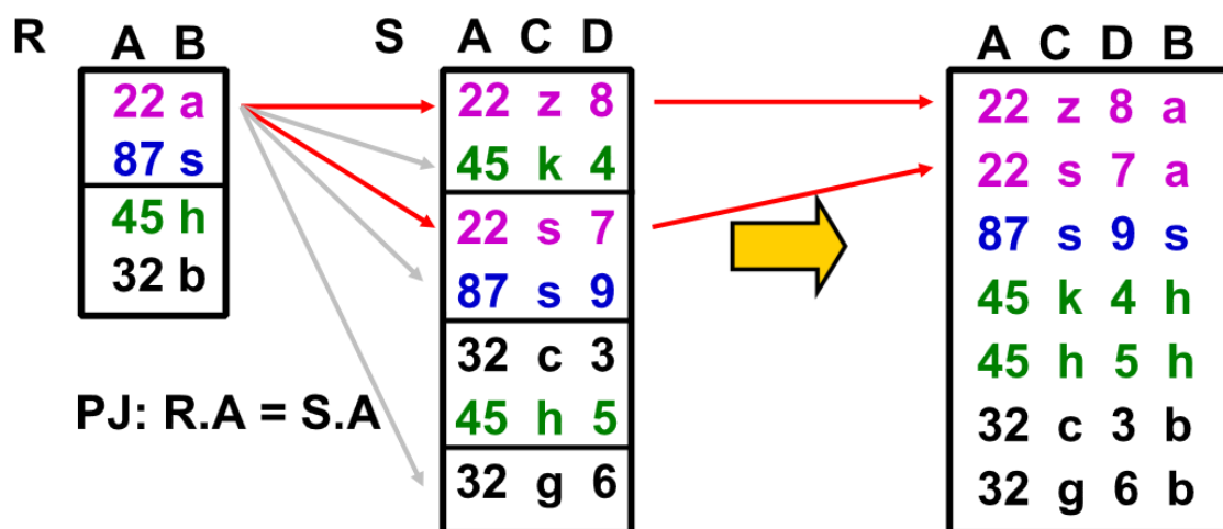
Figura 69: Esempio di nested loop join
