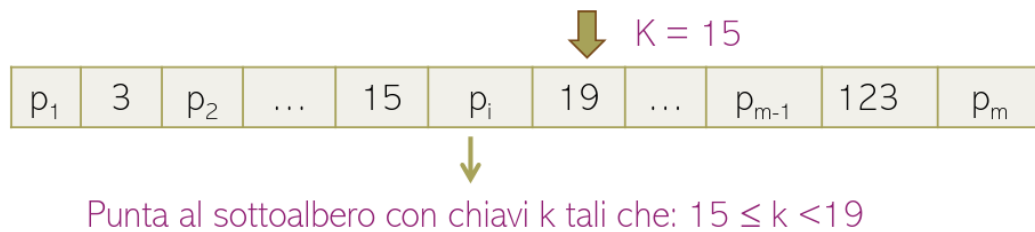
Figura 48: Ricerca di una tupla con chiave di ricerca K in un B+-Tree
