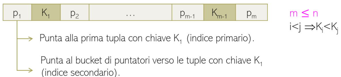
Figure 43: Struttura di un nodo foglia di un B+-Tree con fan-out = n
