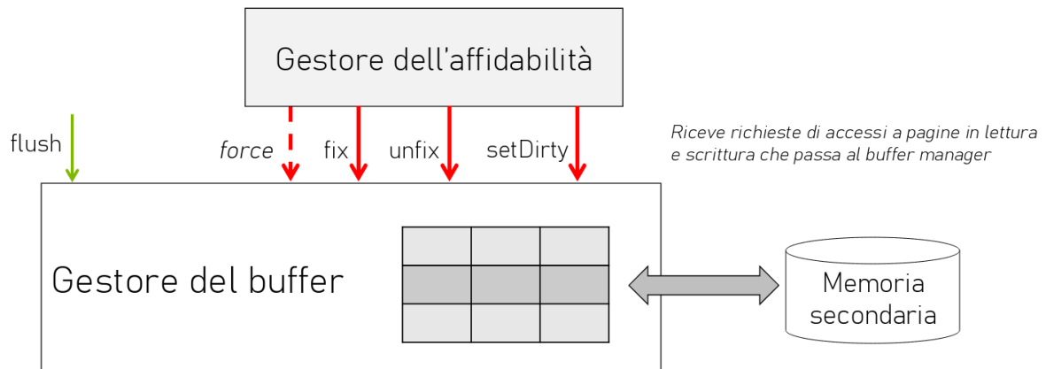
Figura 32: Gestore dell'affidabilità nell'architettura di un DBMS
