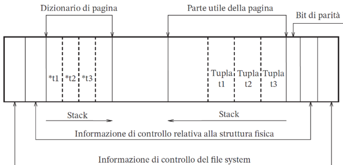
Figura 34: Organizzazione di una pagina
