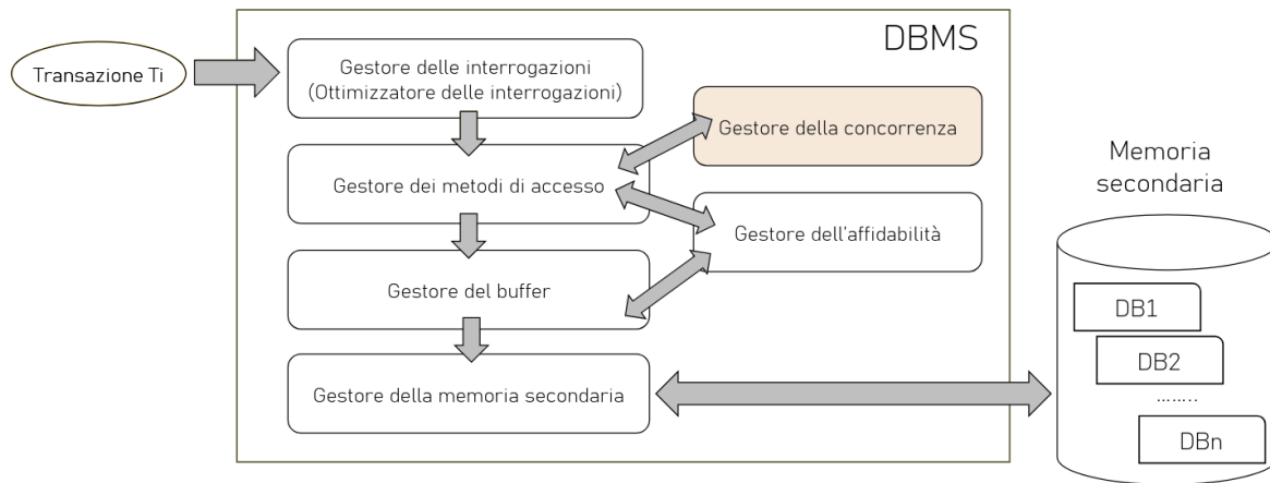
Figura 56: Gestore della concorrenza nell'architettura di un DBMS
