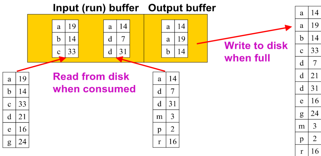
Figura 68: Esempio di utilizzo dei buffer
