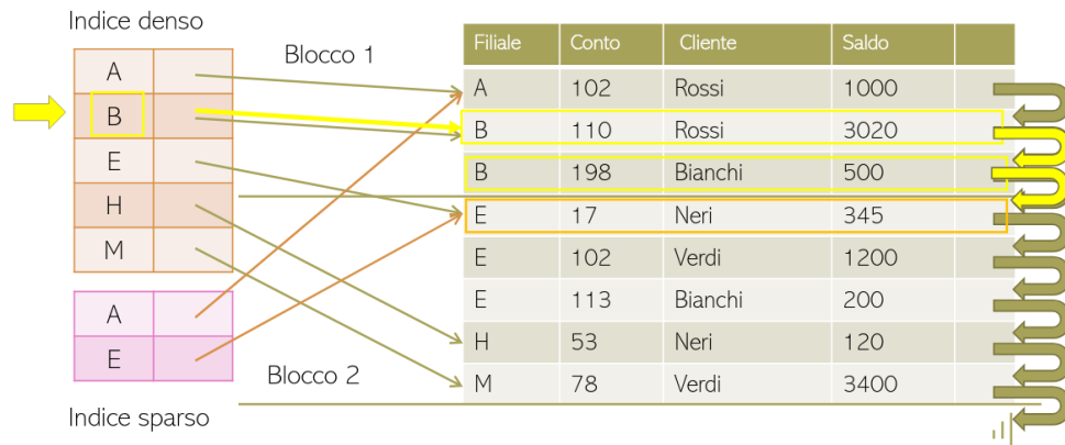
Figura 40: Esempio di ricerca con indice primario denso
