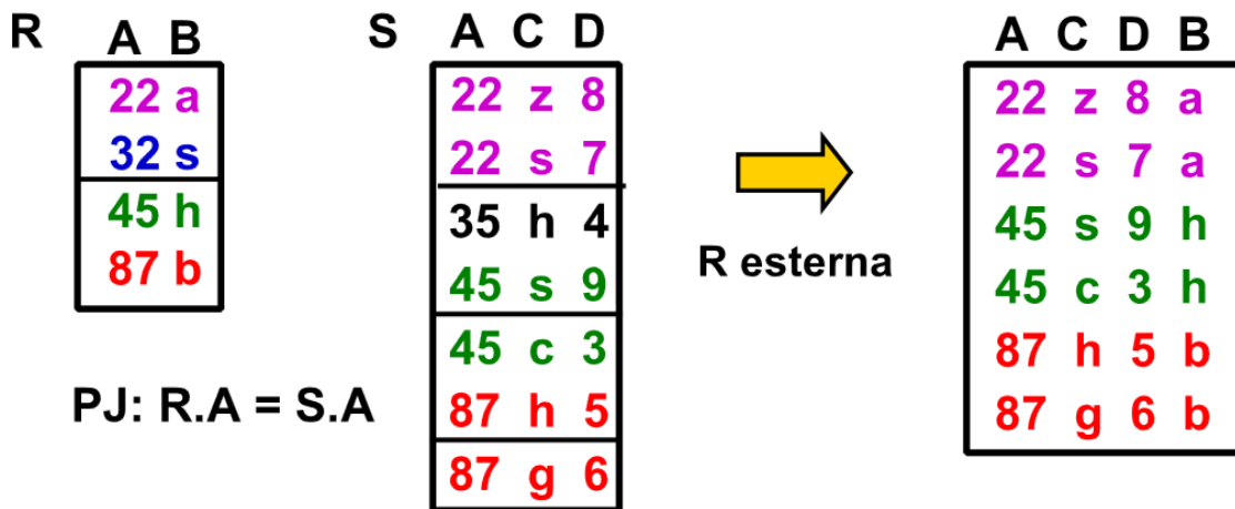
Figura 72: Esempio di merge scan join
