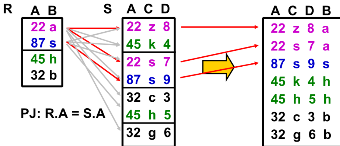
Figura 71: Esempio di block nested-loop join
