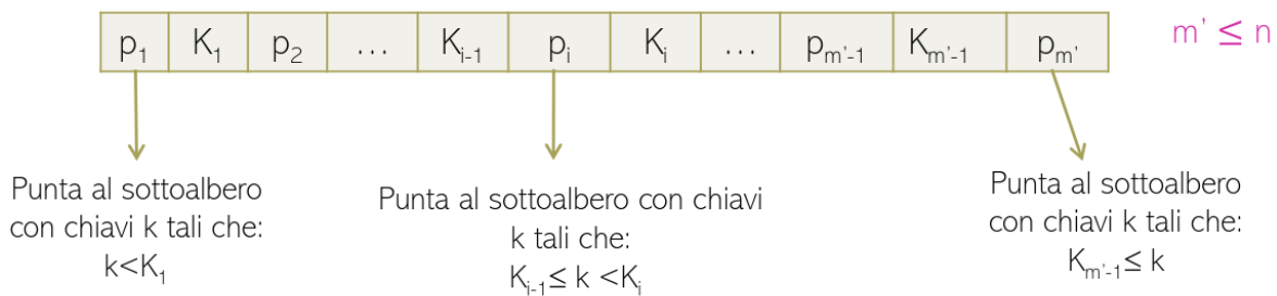
Figura 45: Struttura di un nodo intermedio di un B+-Tree con fan-out = n
