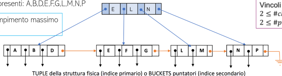
Figura 47: Esempio di B+-Tree con vincolo di riempimento massimo
