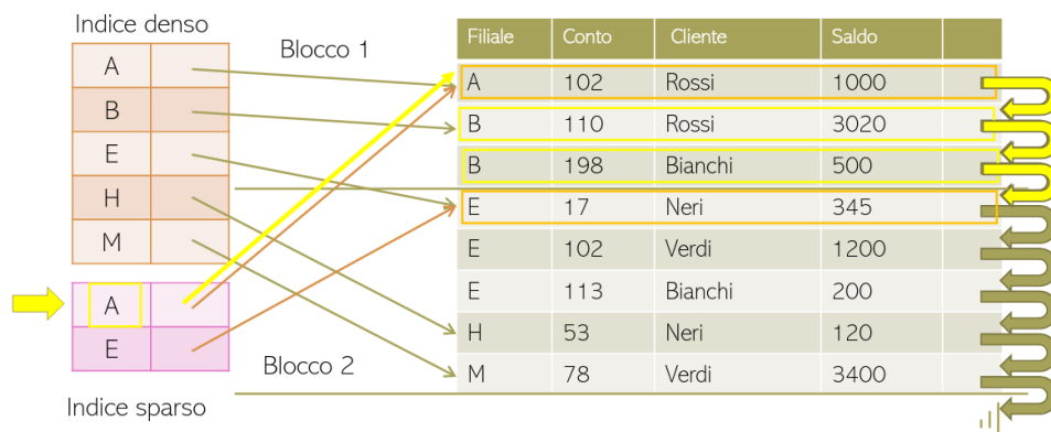
Figura 41: Esempio di ricerca con indice primario sparso
