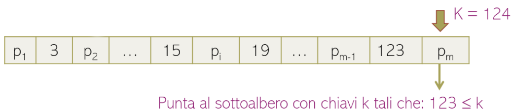
Figura 49: Ricerca di una tupla con chiave di ricerca K in un B+-Tree quando il più piccolo valore di chiave maggiore di K non esiste
