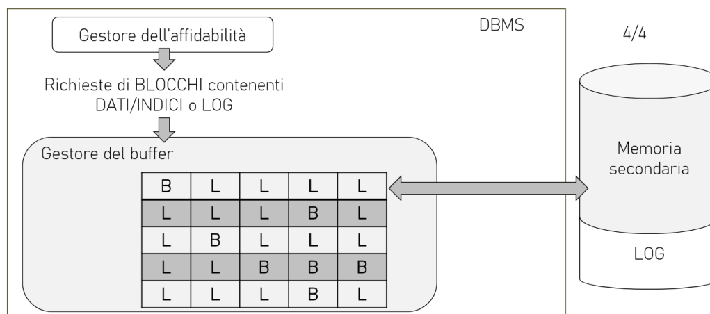
Figura 7: Gestore dell'affidabilità di un DBMS
