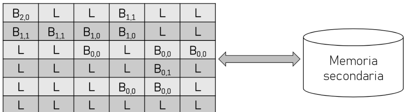
Figura 31: Gestione delle pagine del buffer
