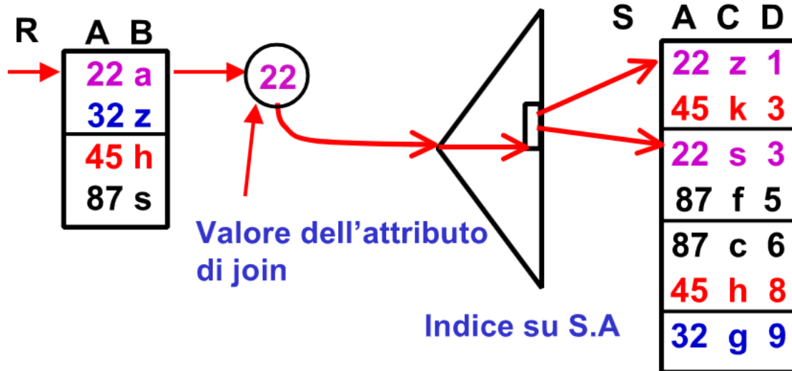
Figura 70: Esempio di nested loop join con indice
