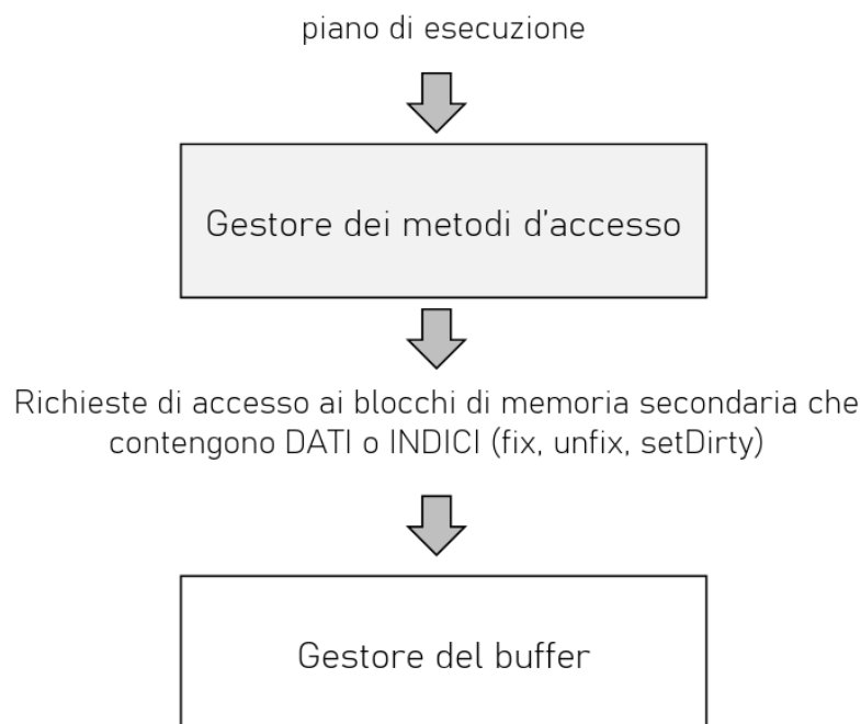
Figura 33: Gestore dei metodi di accesso nell'architettura di un DBMS
