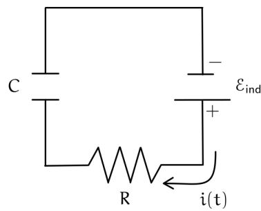
Figura 195: Schema del circuito mobile di Faraday con condensatore
