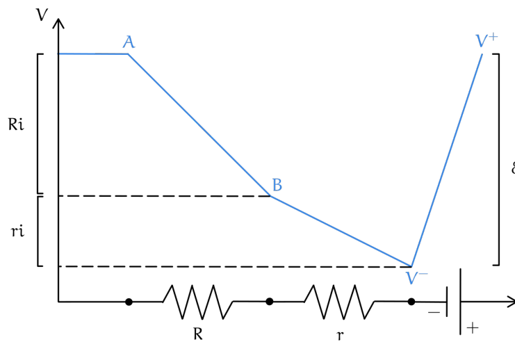
Figura 101: Grafico della tensione
