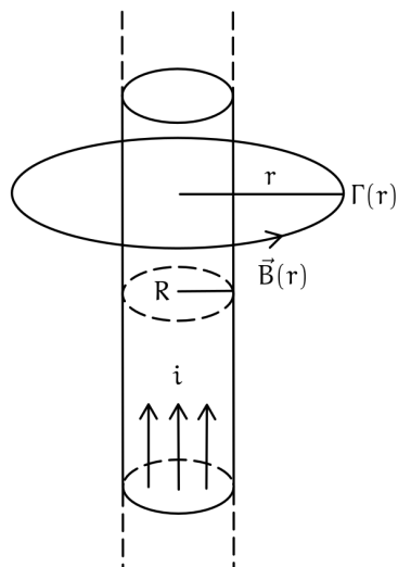
Figura 141: Linea Amperiana
