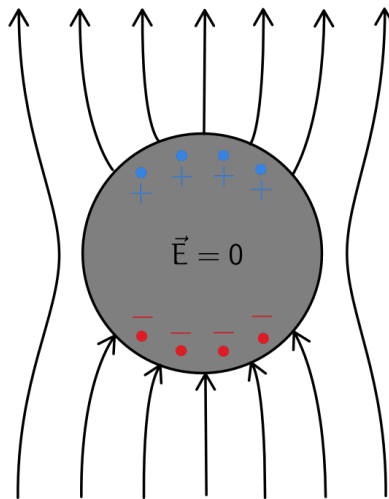
Figura 44: Campo in un conduttore in equilibrio
