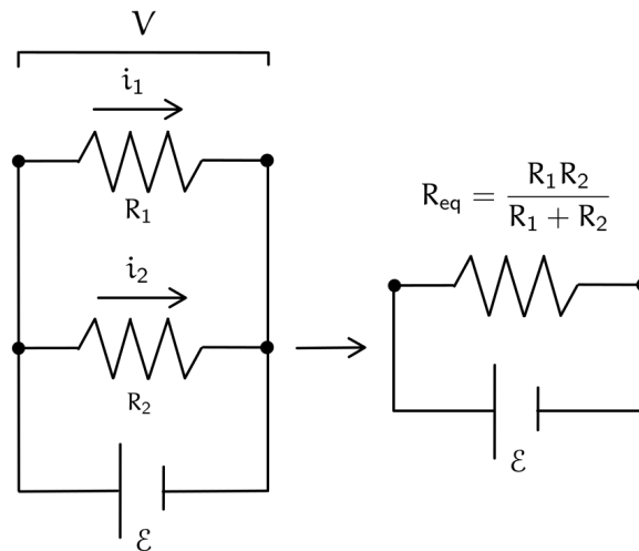
Figura 107: Partitore in corrente
