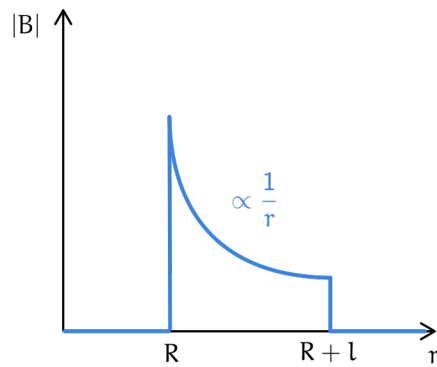
Figura 151: Grafico del campo magnetico
