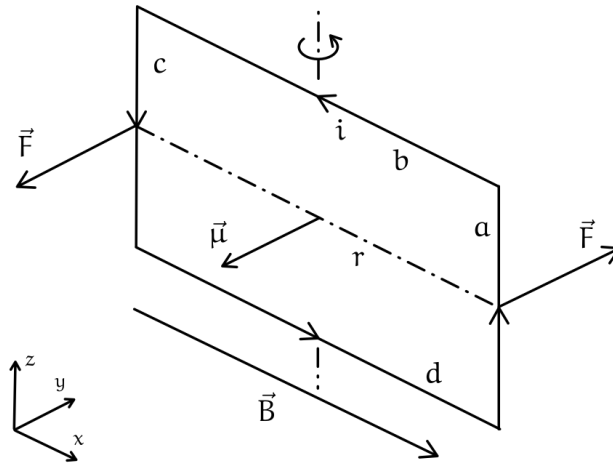
Figura 135: Spira immersa in un campo magnetico
