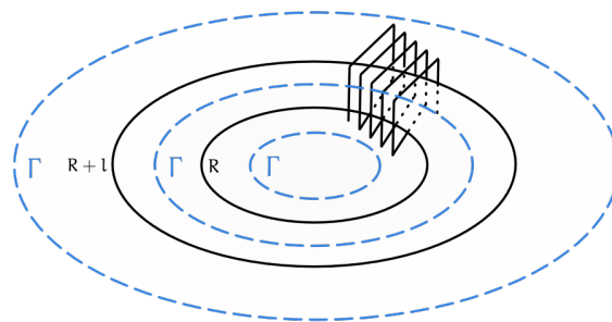
Figura 148: Linea Amperiana toroidale
