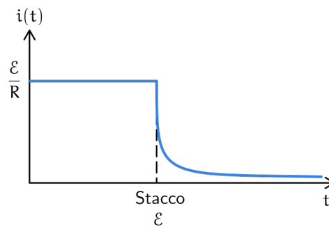
Figura 201: Andamento della corrente durante lo spegnimento
