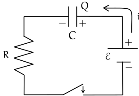
Figura 121: Circuito con condensatore scarico
