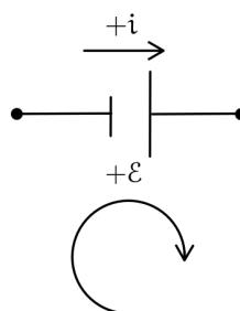
Figura 111: Verso del generatore nella maglia
