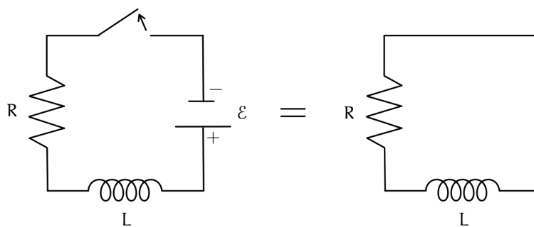
Figura 200: Circuito RL di spegnimento
