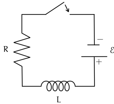
Figura 199: Circuito RL
