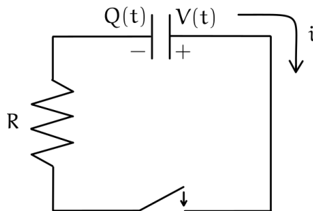
Figura 119: Corrente che scorre dal + al -
