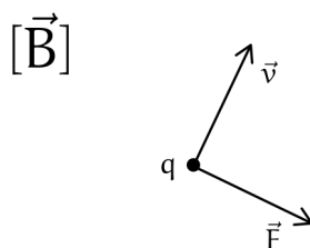
Figura 131: Forza magnetica
