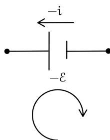
Figura 112: Verso del generatore nella maglia
