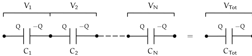
Figura 116: Condensatori in serie
