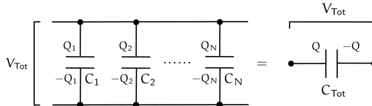
Figura 117: Condensatori in parallelo
