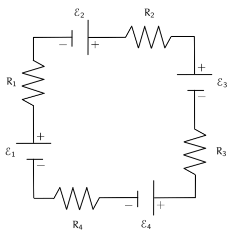
Figura 113: Circuito esempio
