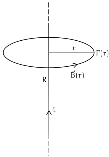
Figura 144: Linea indefinita
