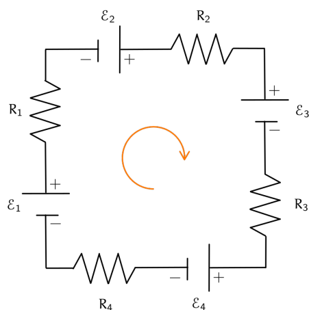
Figura 114: Verso della maglia
