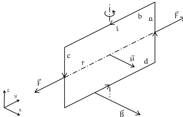
Figura 136: Spira immersa in un campo magnetico
