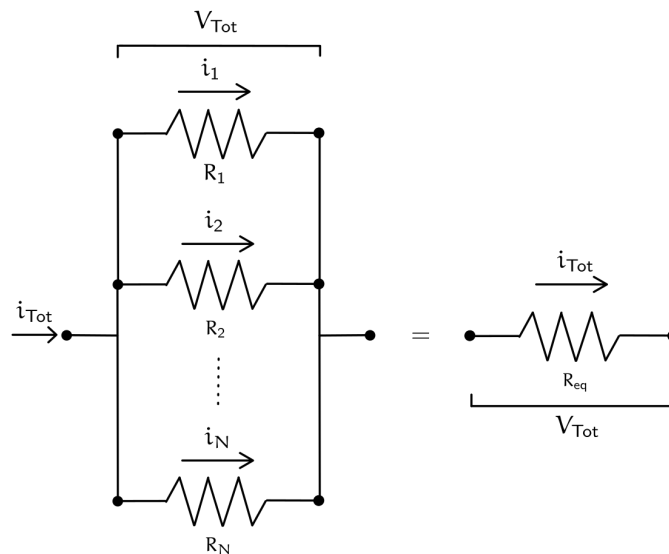
Figura 105: Resistore equivalente in parallelo
