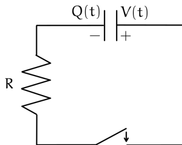
Figura 118: Circuito con condensatore carico
