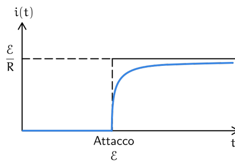
Figura 202: Andamento della corrente durante l'accensione
