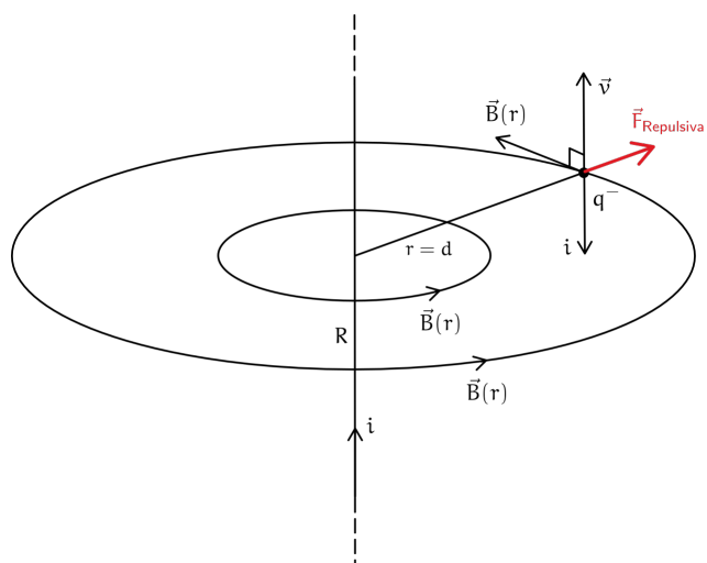
Figura 159: Forza repulsiva
