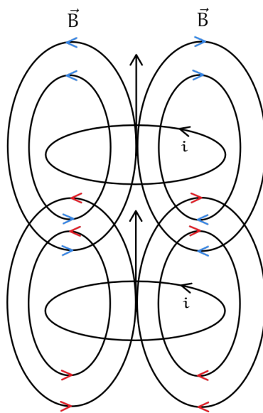
Figura 154: Campo magnetico in più spire
