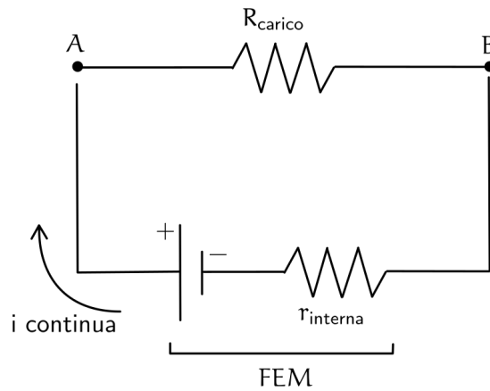
Figura 100: Rete lineare
