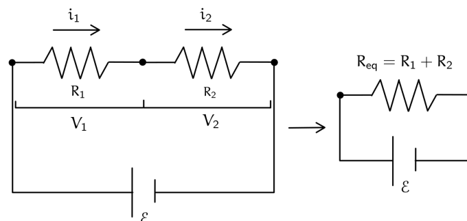
Figura 106: Partitore in tensione
