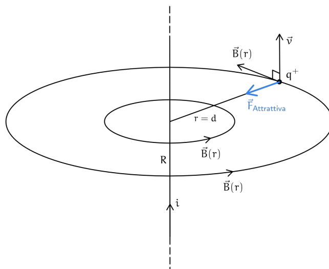
Figura 158: Forza attrattiva
