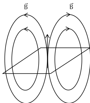
Figura 149: Campo magnetico in una spira
