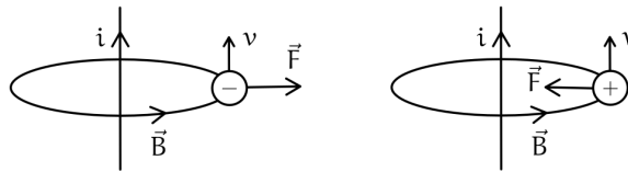
Figura 167: Filo come cariche in movimento
