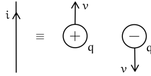
Figura 166: Corrente come cariche in movimento
