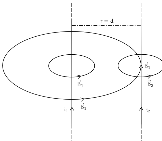
Figura 161: Sul filo i_2 agisce il campo magnetico \vec{B}_1
