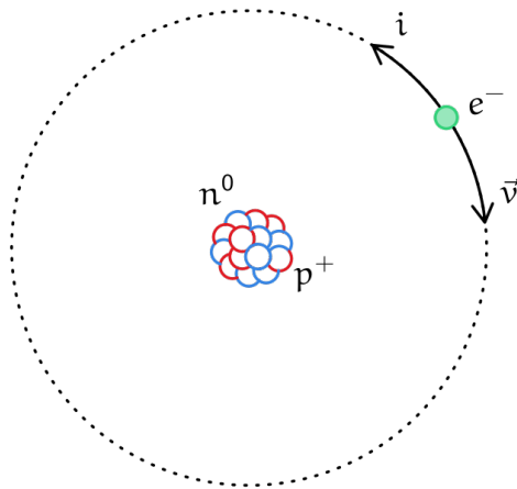
Figura 128: Mirco-corrente Amperiana in un atomo
