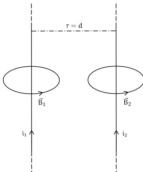
Figura 160: Interazione tra due fili
