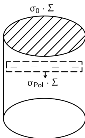
Figura 75: Flusso del campo elettrico in un condensatore piano con dielettrico
