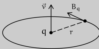
Figura 177: Campo magnetico di una singola carica in moto
