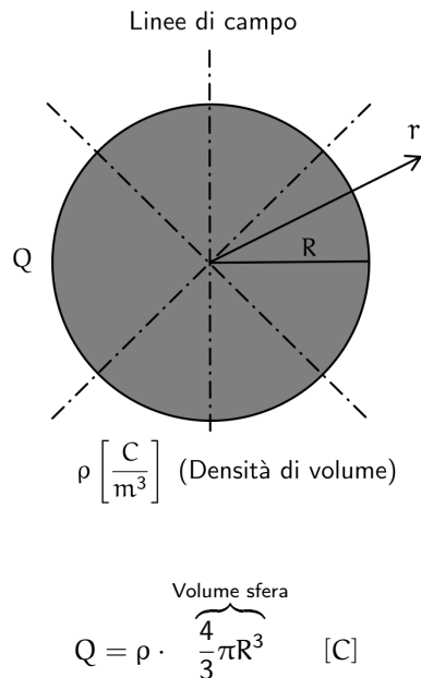
Figura 27: Simmetria sferica di volume
