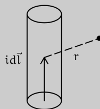
Figura 175: Rappresentazione della prima legge elementare di Laplace
