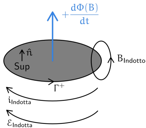
Figura 184: Aumento di flusso
