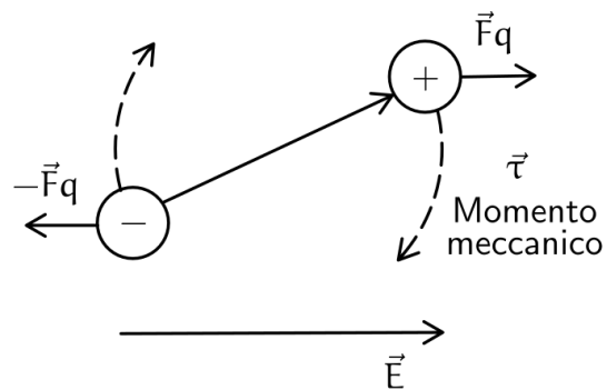
Figura 68: Polarizzazione per orientamento
