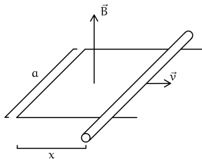
Figura 187: Circuito mobile di Faraday con campo magnetico
