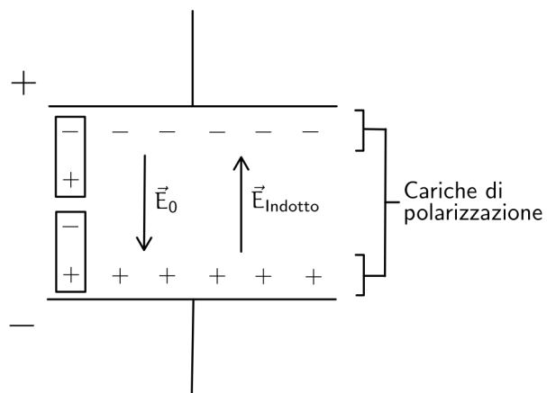
Figura 72: Cariche di polarizzazione
