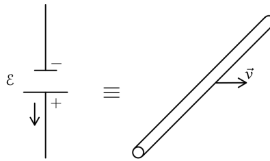
Figura 188: Circuito mobile di Faraday equivalente
