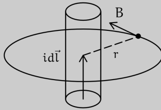
Figura 176: Direzione del campo magnetico
