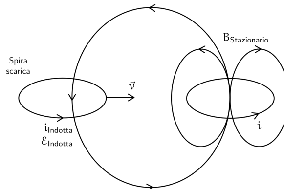
Figura 180: Spira scarica in moto
