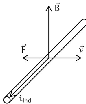
Figura 193: Forza di attrito elettromagnetico
