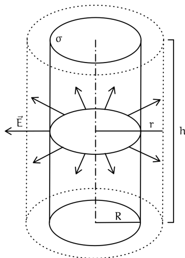
Figura 34: Carica distribuita su un cilindro di raggio R
