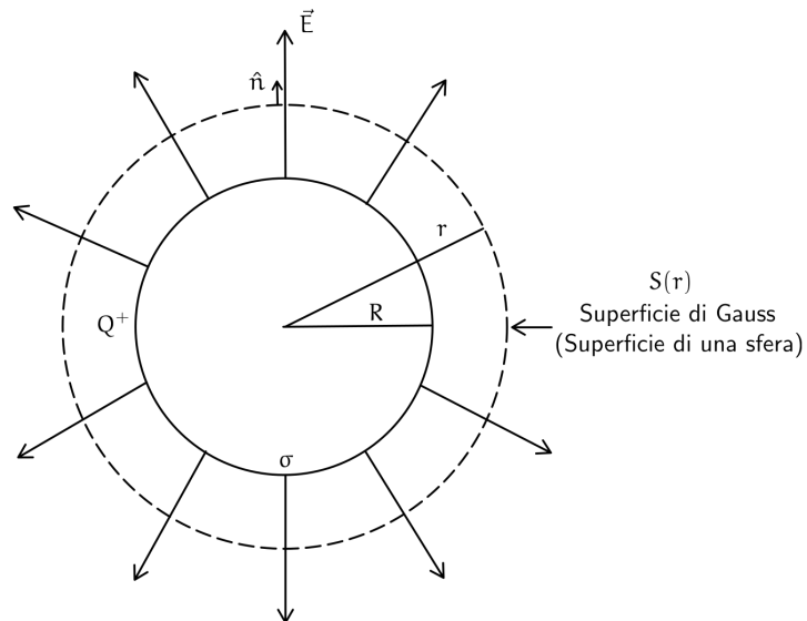
Figura 29: Carica distribuita su una superficie sferica
