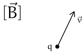
Figura 130: Carica in moto
