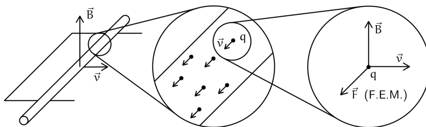
Figura 197: Osservazione del circuito mobile di Faraday
