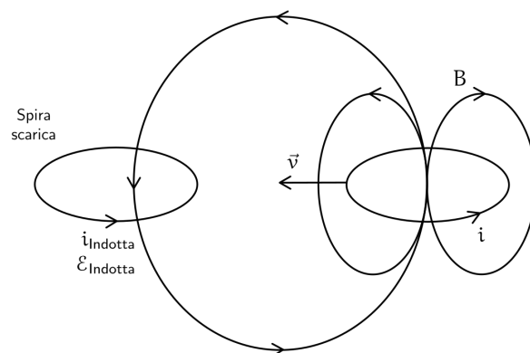
Figura 181: Spira con campo magnetico in moto
