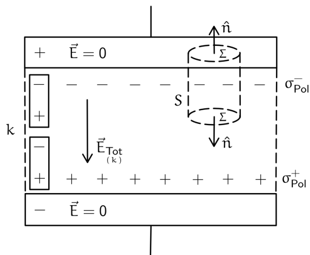
Figura 74: Superficie di Gauss in un condensatore piano con dielettrico
