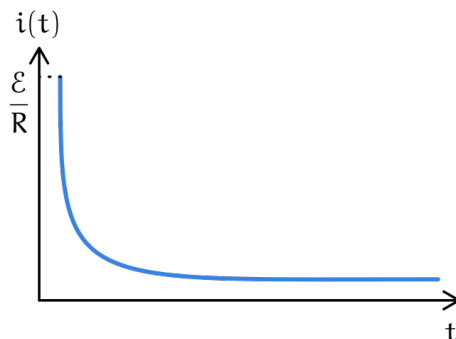
Figura 196: Grafico dell'andamento della corrente
