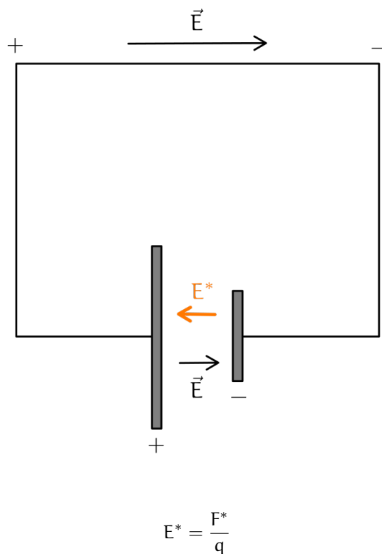
Figura 90: Forza elettromotrice nel dettaglio
