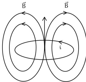
Figura 153: Campo magnetico in una spira
