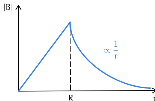
Figura 142: Grafico del campo magnetico
