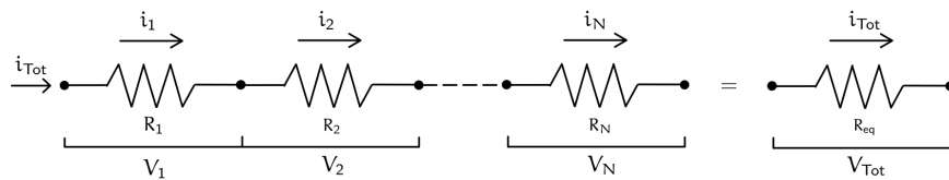
Figura 103: Resistore equivalente in serie
