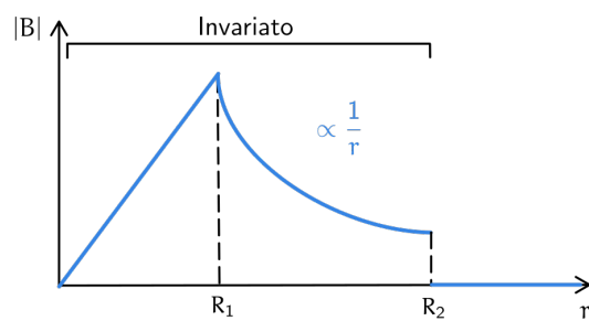
Figura 146: Grafico del campo magnetico
