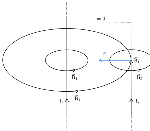
Figura 162: Forza sul filo i_2
