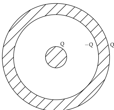
Figura 53: Conduttore con cavità sferica carica
