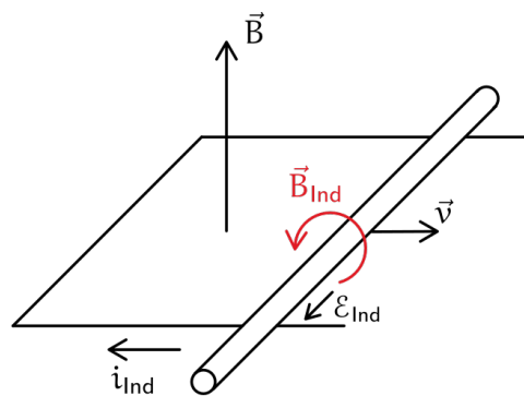
Figura 191: Forza elettromotrice indotta
