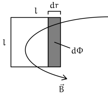
Figura 173: Elemento di superficie della spira
