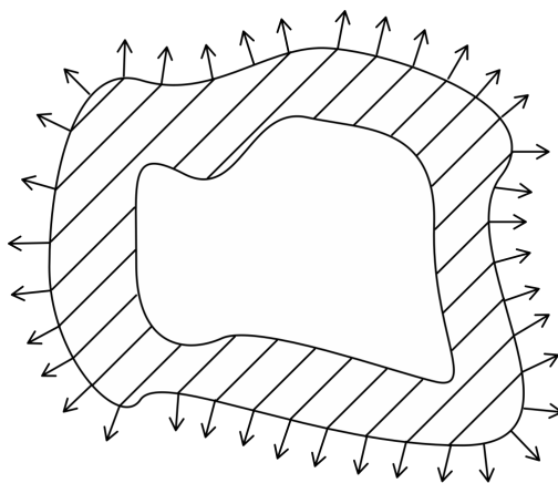
Figura 48: Linee di campo in un conduttore con cavità
