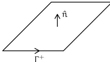
Figura 189: Orientamento del circuito mobile di Faraday
