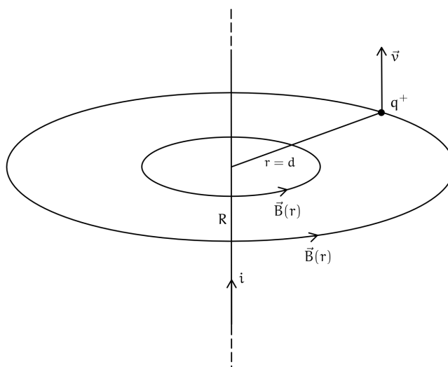
Figura 157: Carica e filo
