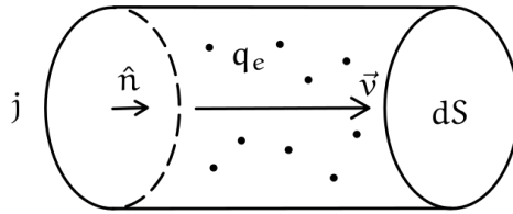
Figura 93: Densità di corrente al livello microscopico
