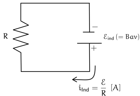
Figura 192: Schema del circuito mobile di Faraday
