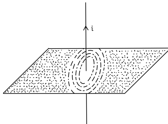
Figura 127: Esperimento di Ørsted
