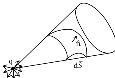
Figura 25: Flusso di una carica puntiforme
