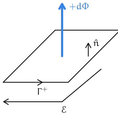
Figura 190: Verso della forza elettromotrice indotta
