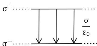
Figura 41: Linee di campo tra due piani
