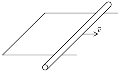
Figura 186: Circuito mobile di Faraday
