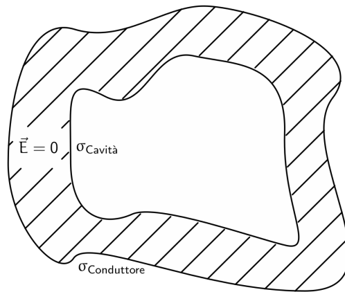
Figura 45: Conduttore con una cavità
