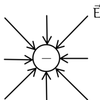
Figura 19: Linee di campo su una carica negativa
