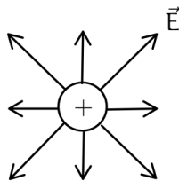
Figura 18: Linee di campo su una carica positiva
