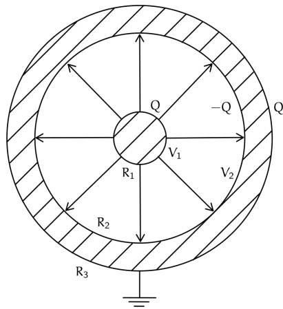
Figura 59: Condensatore sferico
