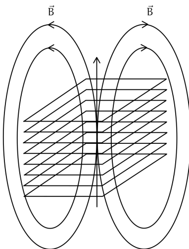
Figura 150: Campo magnetico in più spire
