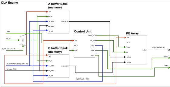
Fig. 2. DLA engine top level.
