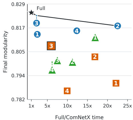
dyn_cora
