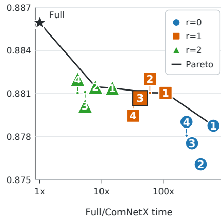
arxivmath
