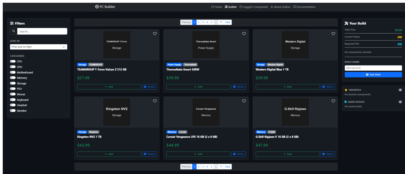
Slika 3. builder.html
