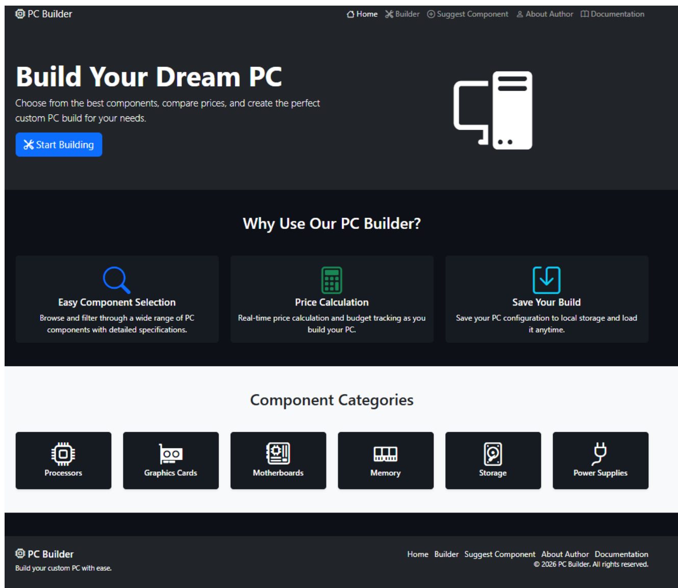
Slika 2. index.html
