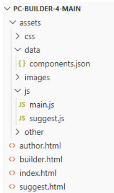
Slika 1. File tree
