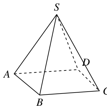
Hình chóp S.ABCD
