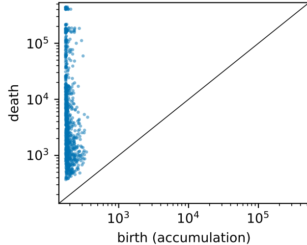
(d) H0 persistence diagram (n=928 H0 features)
