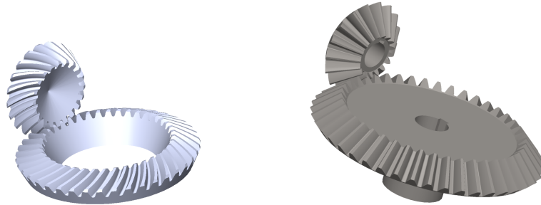
Pignons coniques à dentures hélicoïdales Pignons coniques à dentures droites
