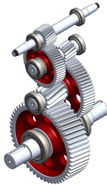
dentures hélicoïdales
