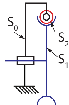
Schéma cinématique
