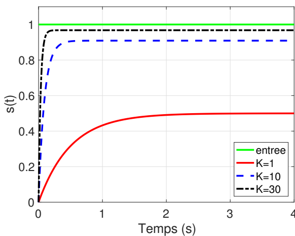
Réponse indicielle 1 er ordre
