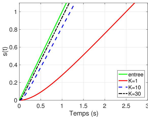
Réponse à une rampe 1 er ordre
