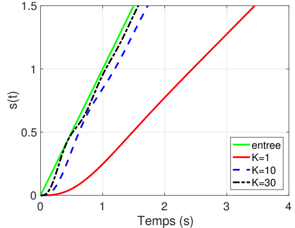
Réponse à une rampe 2 ème ordre
