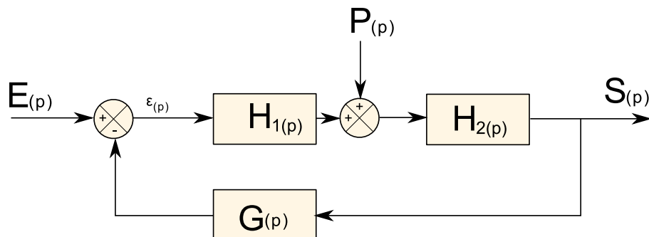
FIGURE 1 – Schéma bloc avec perturbation
