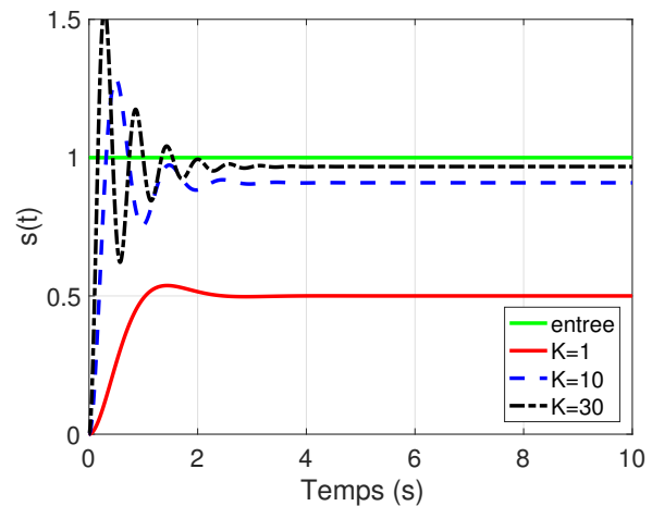
Réponse indicielle 2 ème ordre
